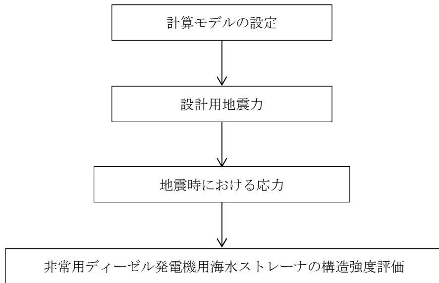
図 2-1 非常用ディーゼル発電機用海水ストレーナの耐震評価フロー
