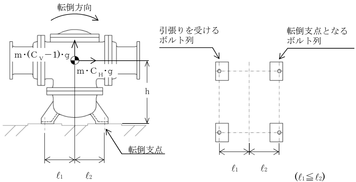
図5-3 計算モデル（長辺方向転倒）
