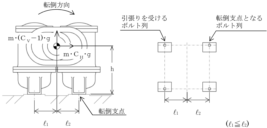
図5-2 計算モデル（短辺方向転倒）
