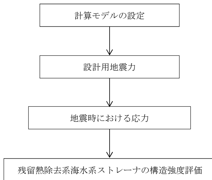
図 2-1 残留熱除去系海水系ストレーナの耐震評価フロー
