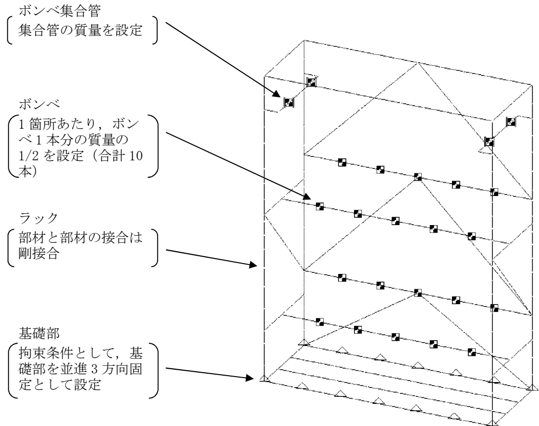
図3-1 解析モデル
