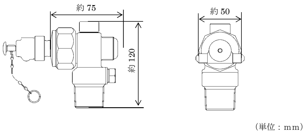
図 2-2 容器弁 外観図
