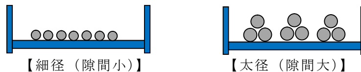
第 3-5 図 ケーブル組合せ
