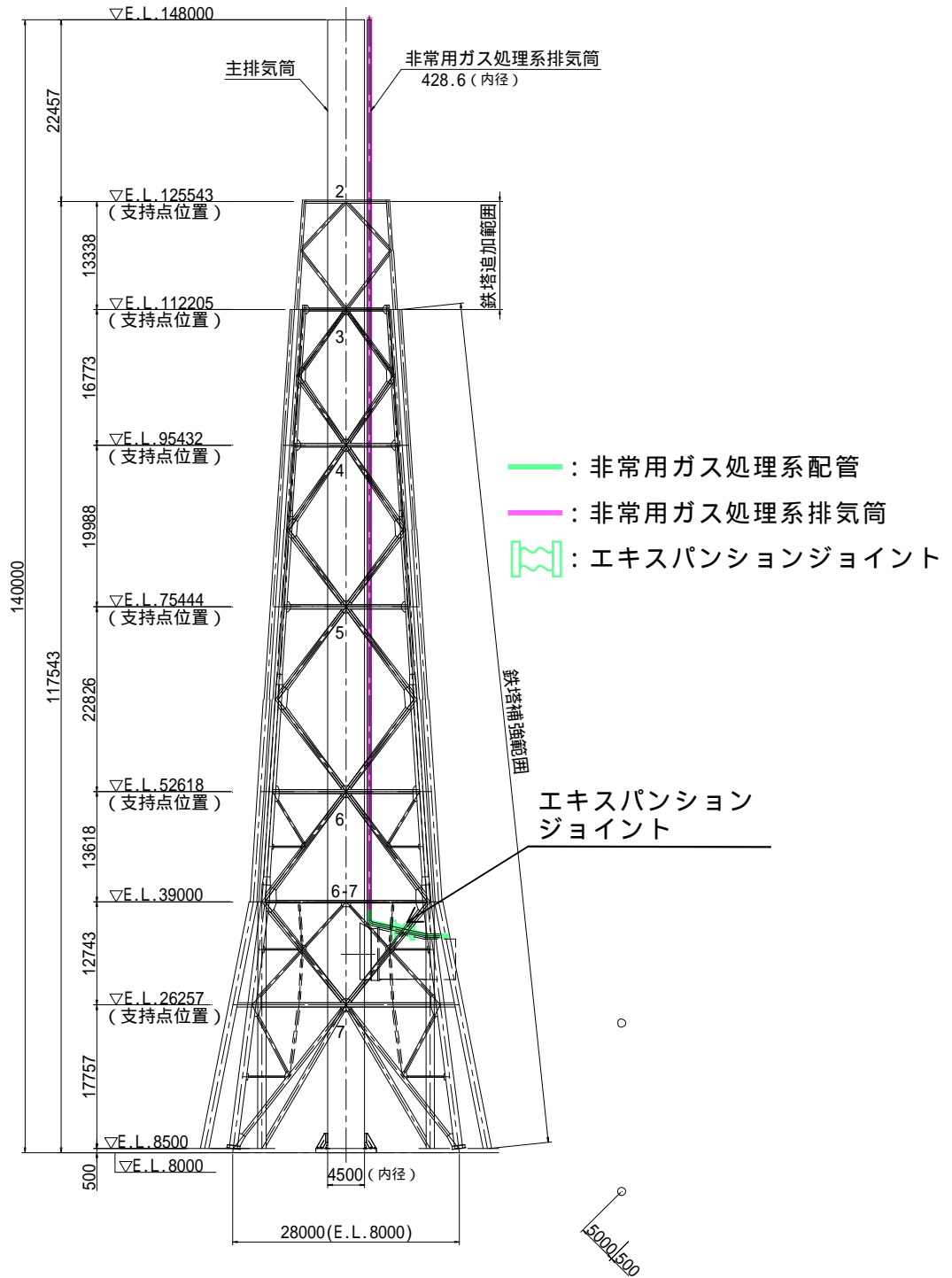
図 6-1-1 エキスパンションジョイントの設置位置
