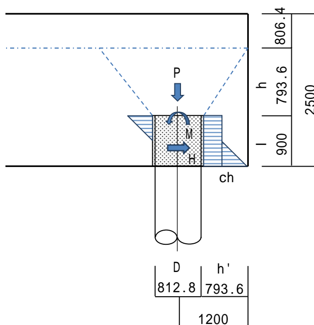
図 5-2-1 杭頭部構造図
