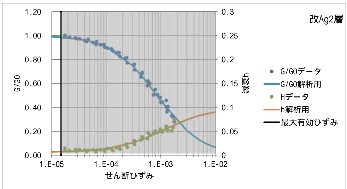
図 2-3-6 地盤物性 ( G/G_0 曲線, h 曲線 ) 改 Ag2 層
