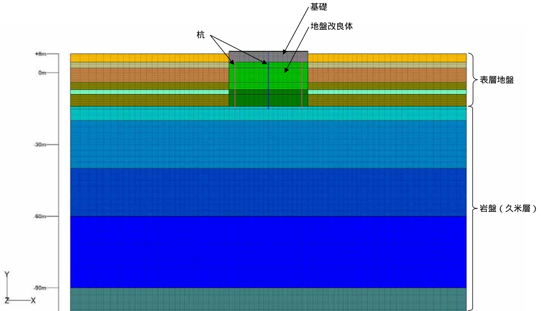
図 2-3-11 2次元 FEM モデル図 (改良体周辺)
