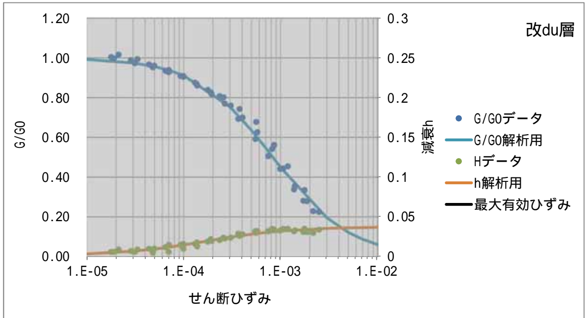
図 2-3-5 地盤物性 ( G/G_0 曲線, h 曲線 ) 改 du 層
