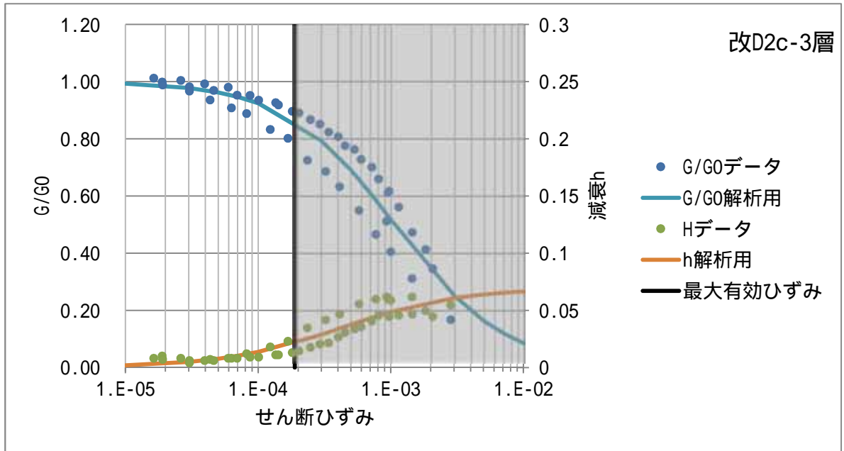
図 2-3-7 地盤物性 ( G/G_0 曲線, h 曲線 ) 改 D2c-3 層
