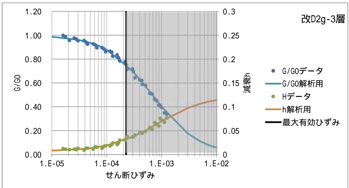
図 2-3-8 地盤物性 ( G/G_0 曲線, h 曲線 ) 改 D2g-3 層
