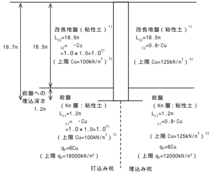
図 4-3-1 杭の鉛直支持力及び引抜き抵抗力の算定プロセス
