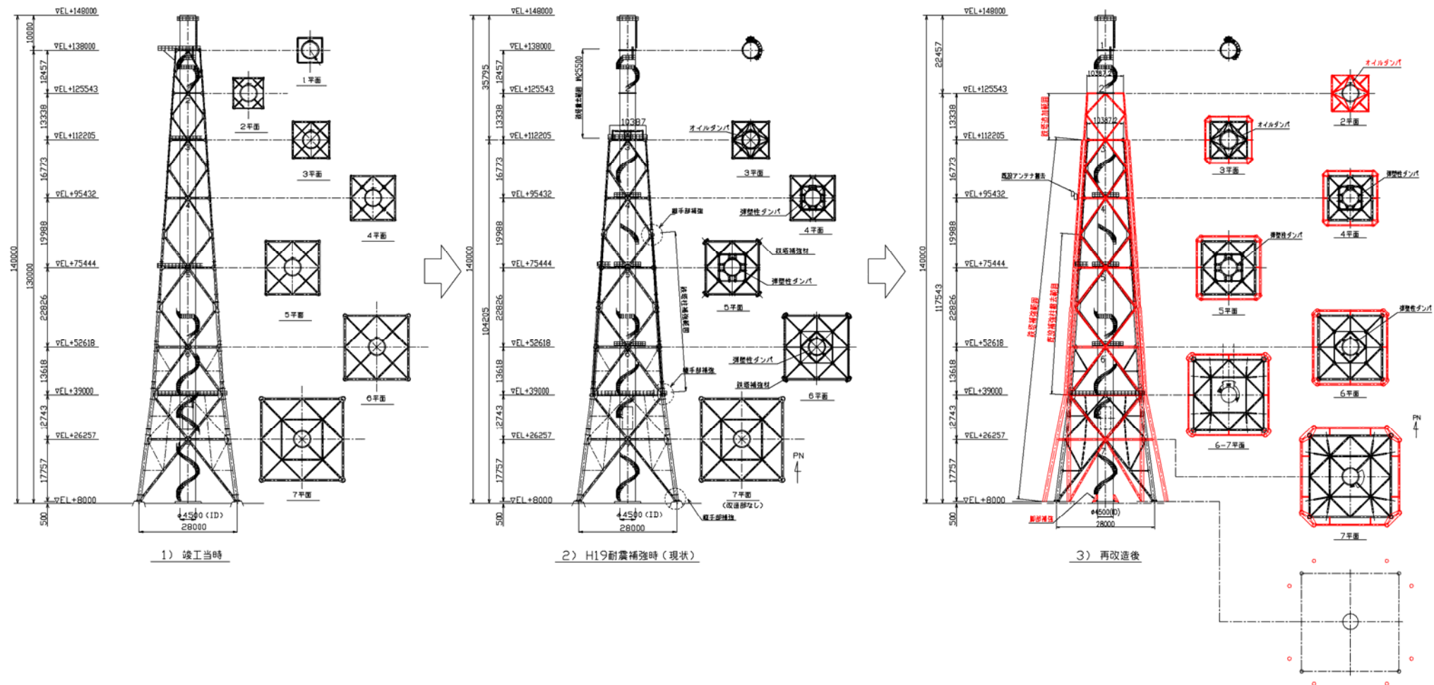
図 1-2-1 主排気筒上部構造の改造履歴
