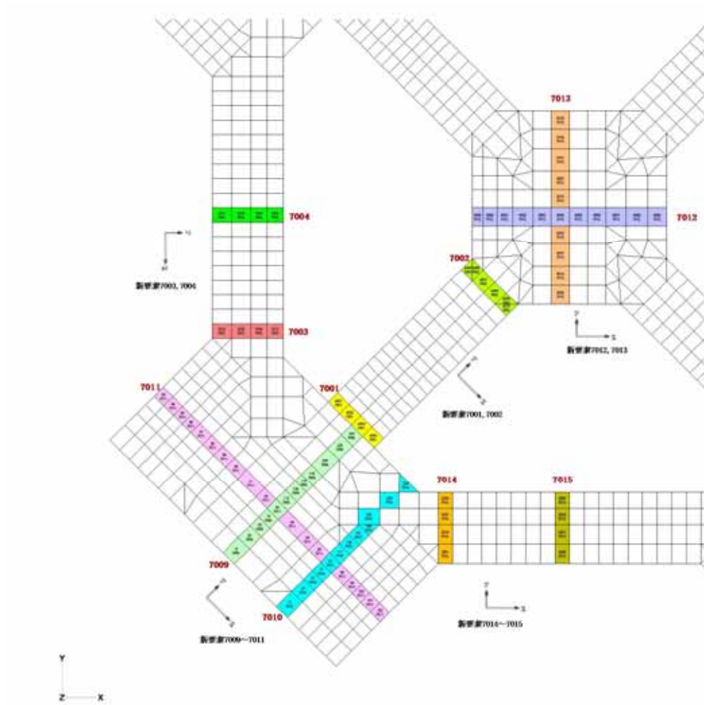
図 4-2-2 主排気筒基礎の評価断面算定位置
