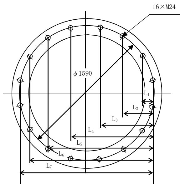
図 3-9 基礎ボルト配置図
