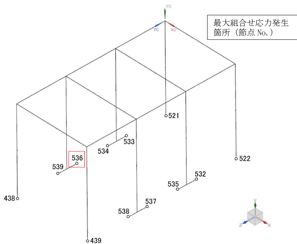
図 5-2 基礎ボルトの最大応力発生箇所（ブレース等非表示モデル図）
