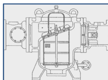
(b) 側面図
