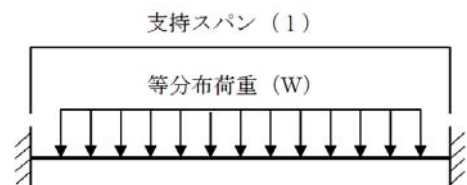
図 3.4-10 タービン建屋 屋根スラブ 評価モデル図(両端固定梁)
