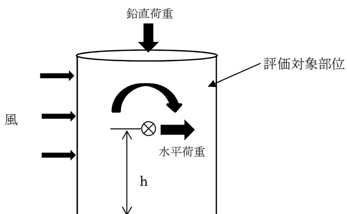
図 3-3 1 質点系モデル図（原動機フレーム）
