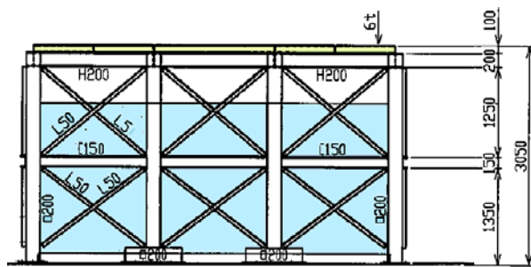
(c) 側面図 (A-A 矢視)
