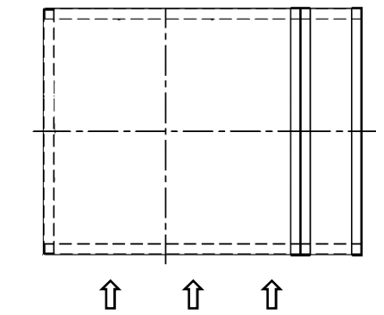
(a) 上面図
