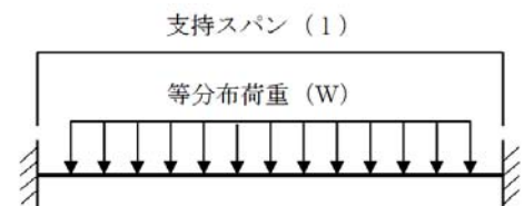
図 3.4-6 原子炉建屋付属棟 屋根スラブ 評価モデル図(両端固定梁)
