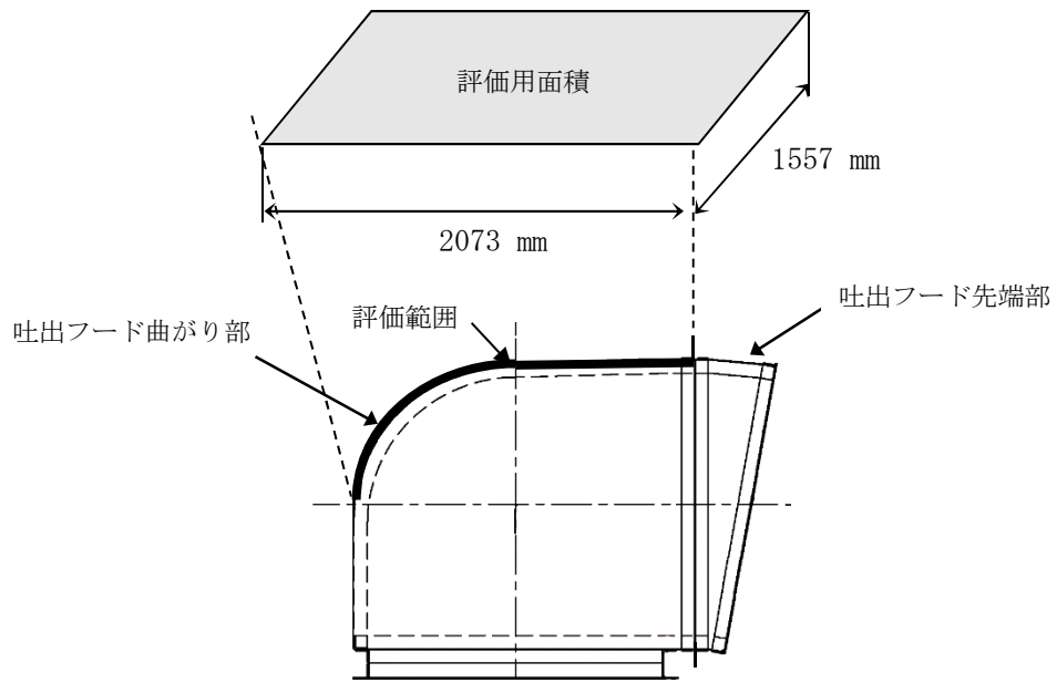
(b) 側面図
