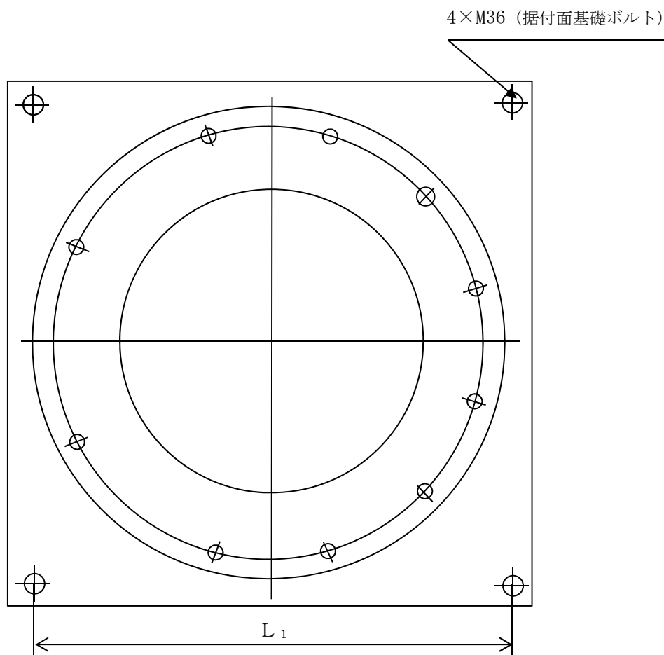
図 3-8 据付面基礎ボルト*の配置図
