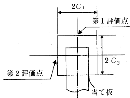
図 3-9 胴の評価点
