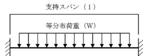
図 3.4-1 原子炉建屋原子炉棟 屋根スラブ 評価モデル図(両端固定梁)
