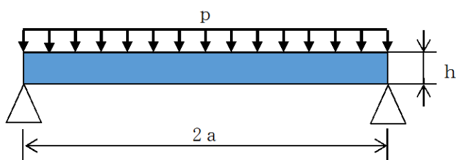
図 3-3 等分布荷重による評価に用いるモデル図
