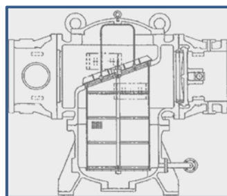
(b) 側面図
