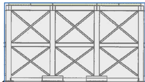
(b) 側面図
