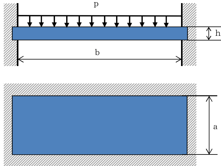
図 3-3 等分布荷重による評価に用いるモデル図
