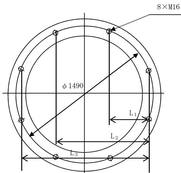
図 3-8 吐出フード取付ボルト配置図
