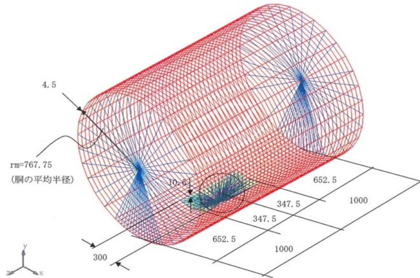
図 3-8 3次元FEMモデル図
