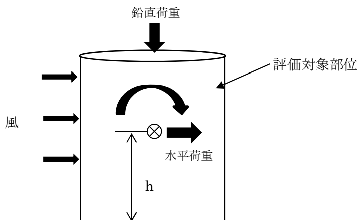
図 5.5.1-1 1 質点系モデル図 (原動機フレーム)
