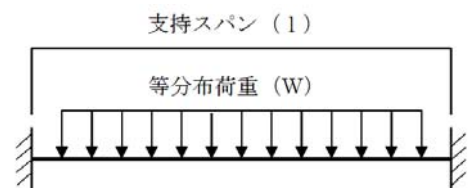
図 3.4-15 使用済燃料乾式貯蔵建屋 屋根スラブ 評価モデル図(両端固定梁)
