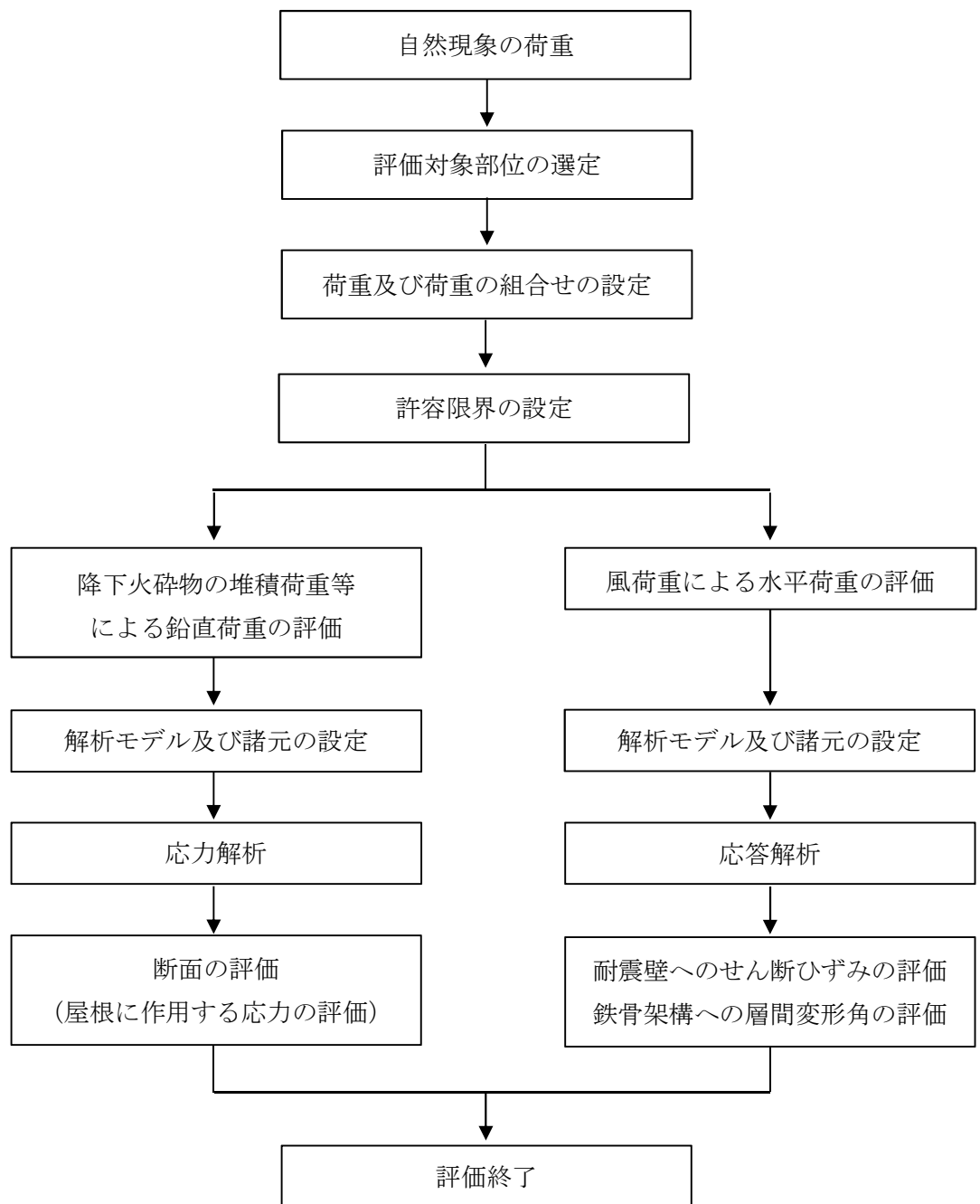
図 2-12 強度評価フロー
