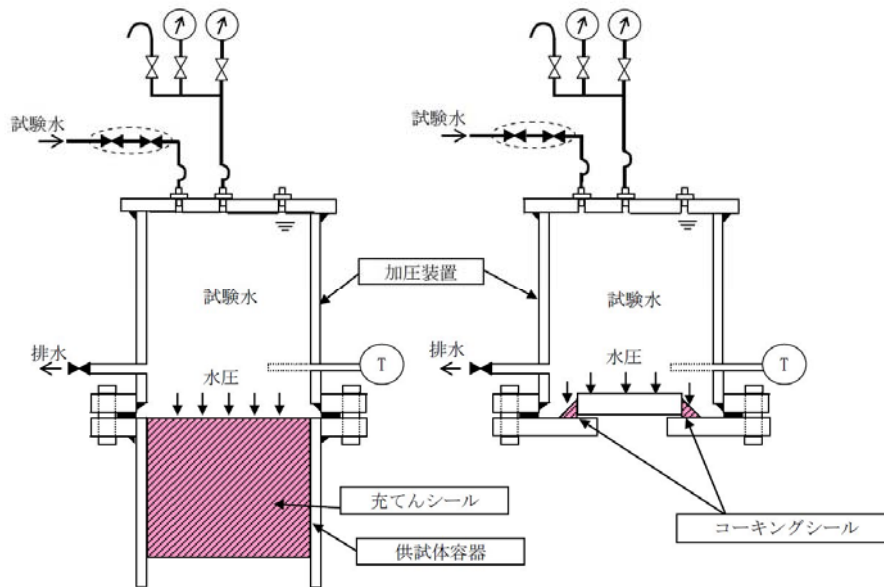
図 3-1 シール材の水圧試験の概要
