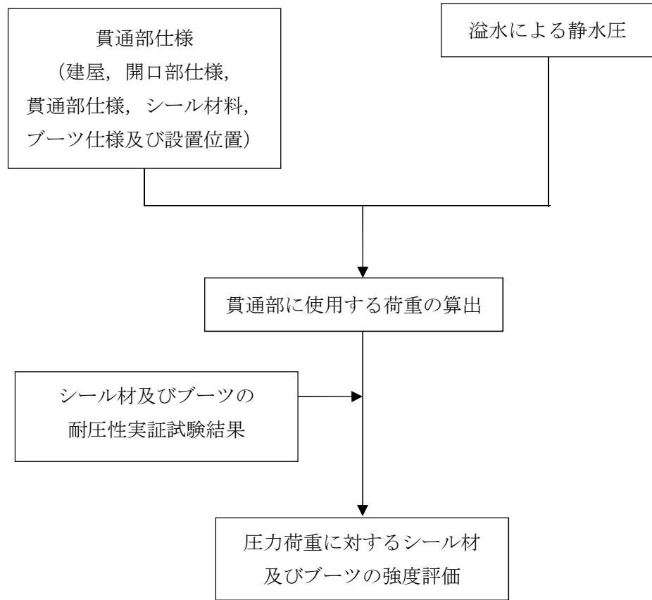
図 2-2 シール材及びブーツの強度評価フロー
