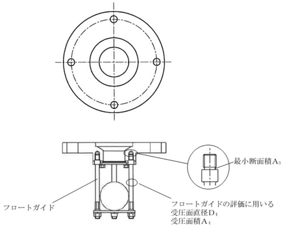
図 5-20 フロートガイドの強度評価に用いる受圧面直径及び断面積
