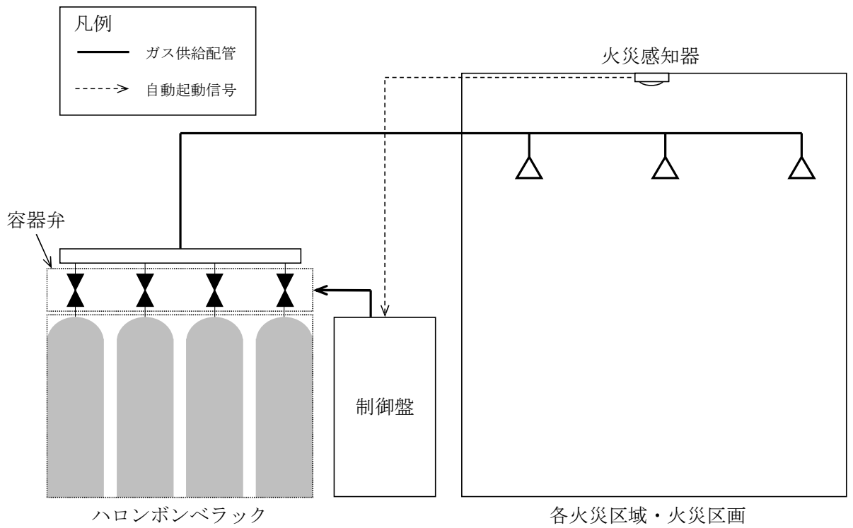
第5-5図 ハロゲン化物自動消火設備（全域） 自動起動信号
