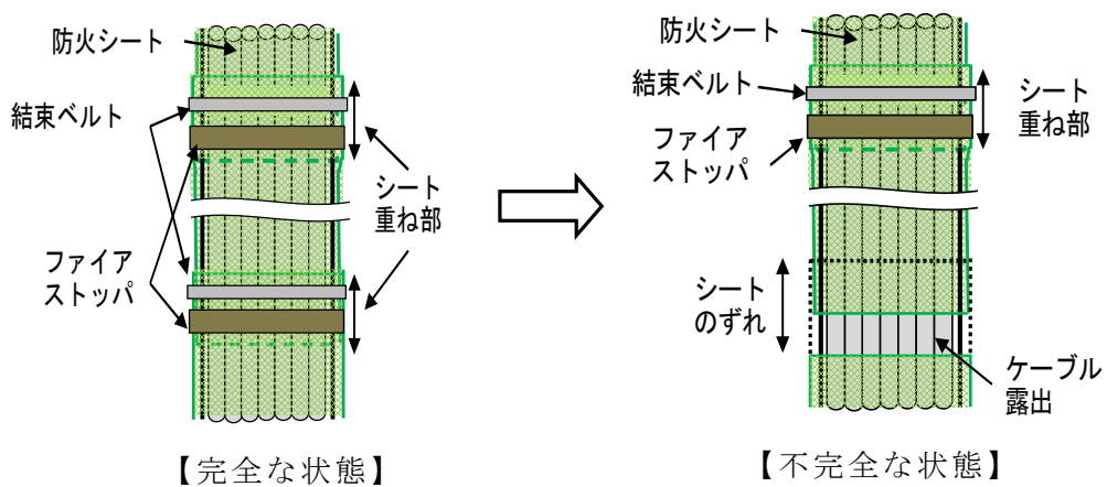
第 5-1 図 防火シートつなぎ部のずれ（複合体正面）
