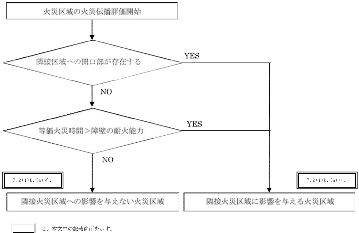
第7-1図 火災伝播評価手順の概要フロー
