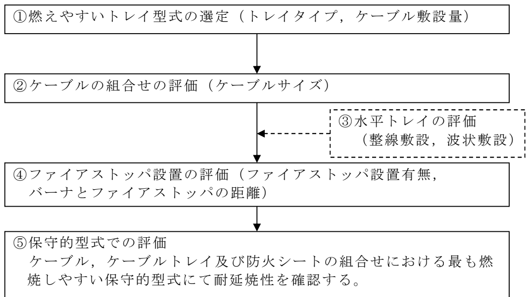
第 3-2 図 実機模擬試験の実施に係る保守的型式の決定フロー
