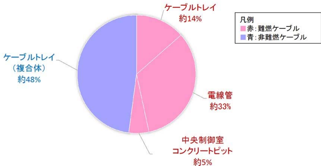
第 4 図 難燃ケーブルと非難燃ケーブル (複合体) の長さの割合
