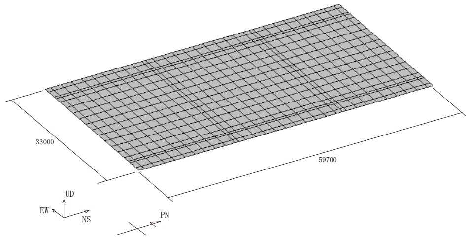
(b) 基礎スラブ
