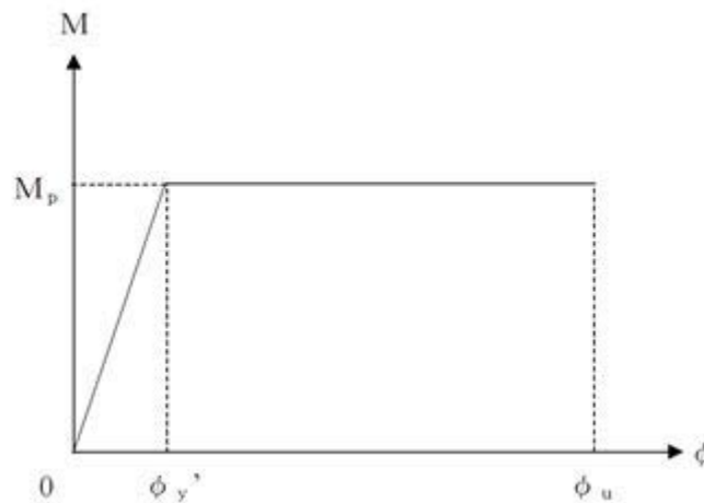
図 3-6 杭の M - \phi 関係
