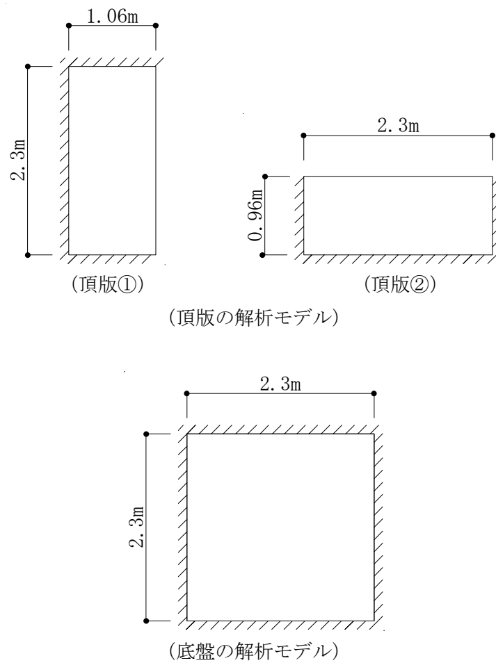
図 4-1 解析モデル
