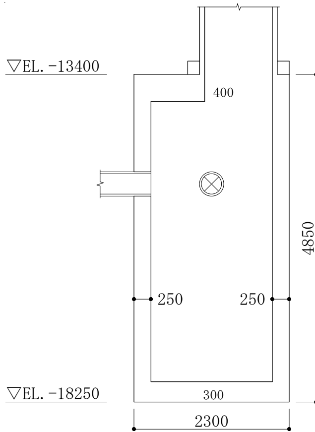
図 2-4 集水ピットの概略断面図（a-a 矢視/NS 方向断面）
