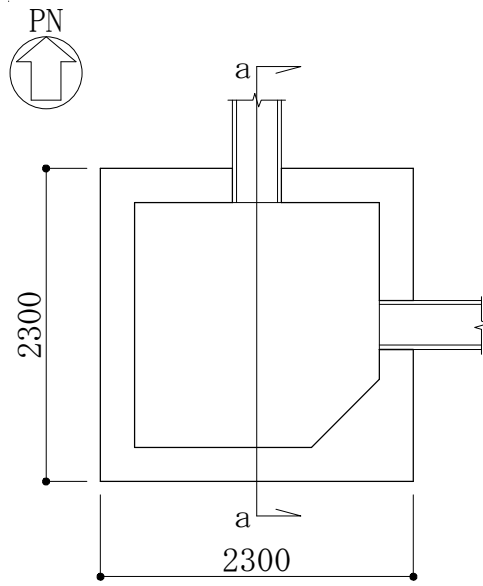
図 2-3 集水ピットの概略平面図（南西隅）
