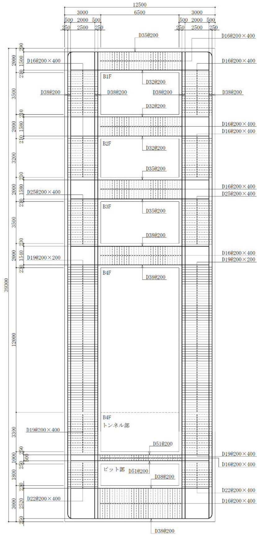
図 4-1 (1) 概略配筋図 (南北方向断面)
