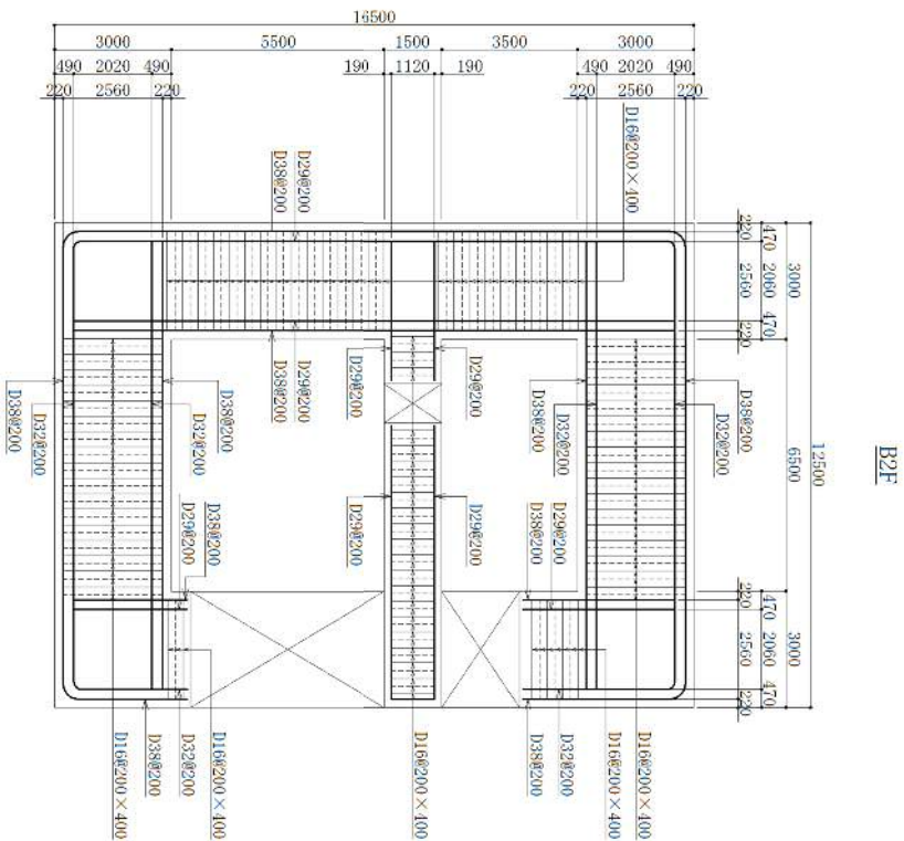
図 4-1 (3) 概略配筋図
