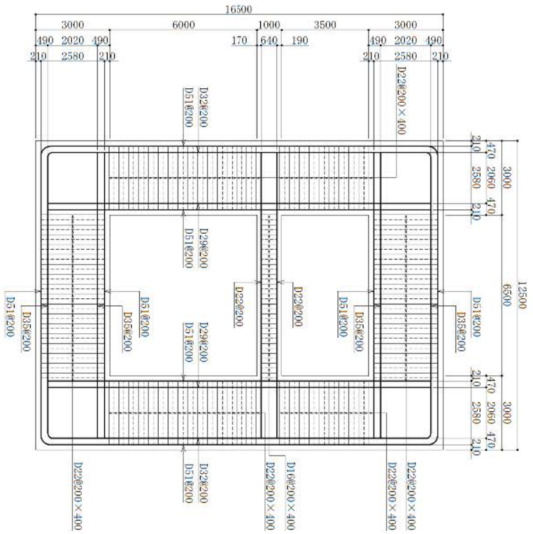
図 4-1 (5) 概略配筋図
