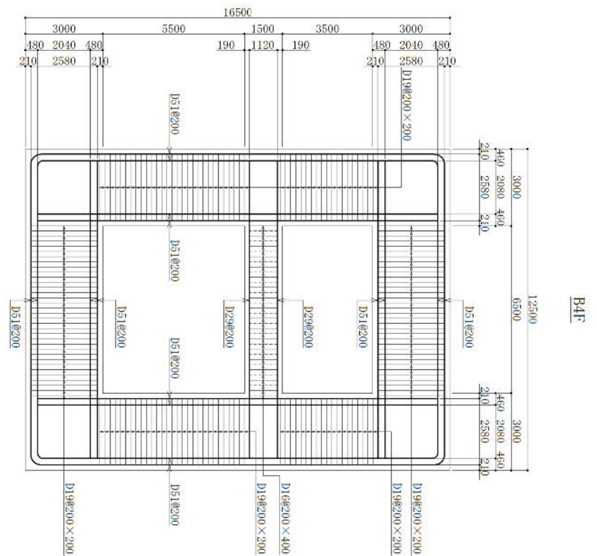
図 4-1 (4) 概略配筋図
