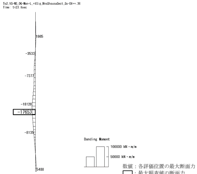
曲げモーメント (kN · m/m)
