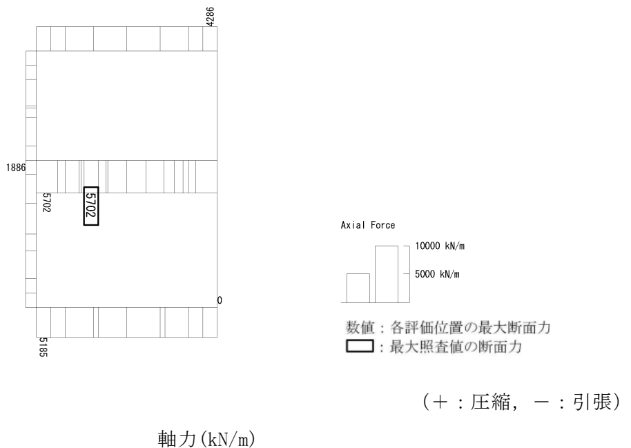
図 3-7 水平断面の曲げ軸力照査における最大照査値の評価時刻での断面力
