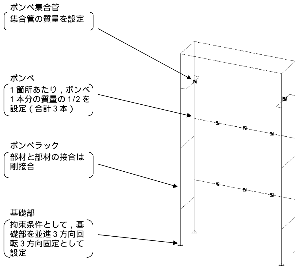
図 3-1 解析モデル
