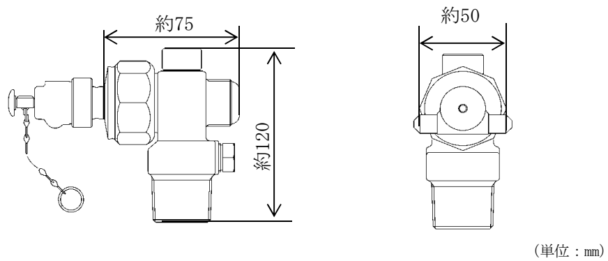
図2-6 容器弁 外観図
