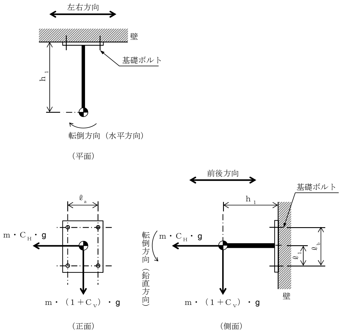
図5-2 熱感知器，煙感知器①，光電分離式煙感知器及び屋外仕様炎感知器 構造強度評価モデル
