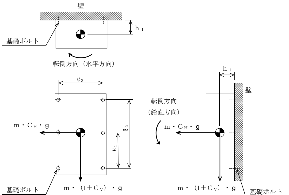
図5-11 壁掛型の構造強度評価モデル
