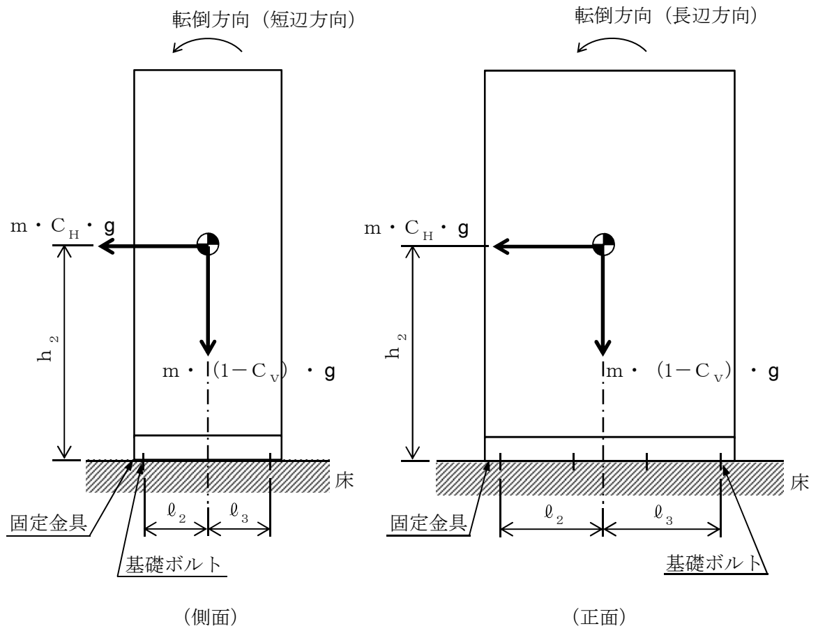
図5-5 煙感知器② 構造強度評価モデル
