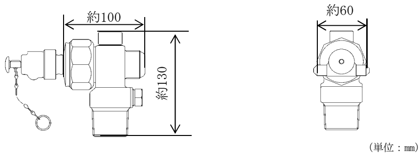
図2-2 容器弁 外観図
