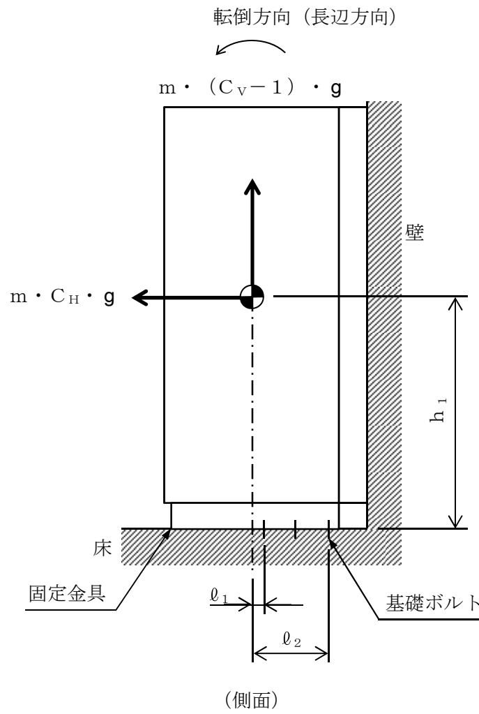
図5-7 火災受信機盤 長辺方向の構造強度評価モデル
