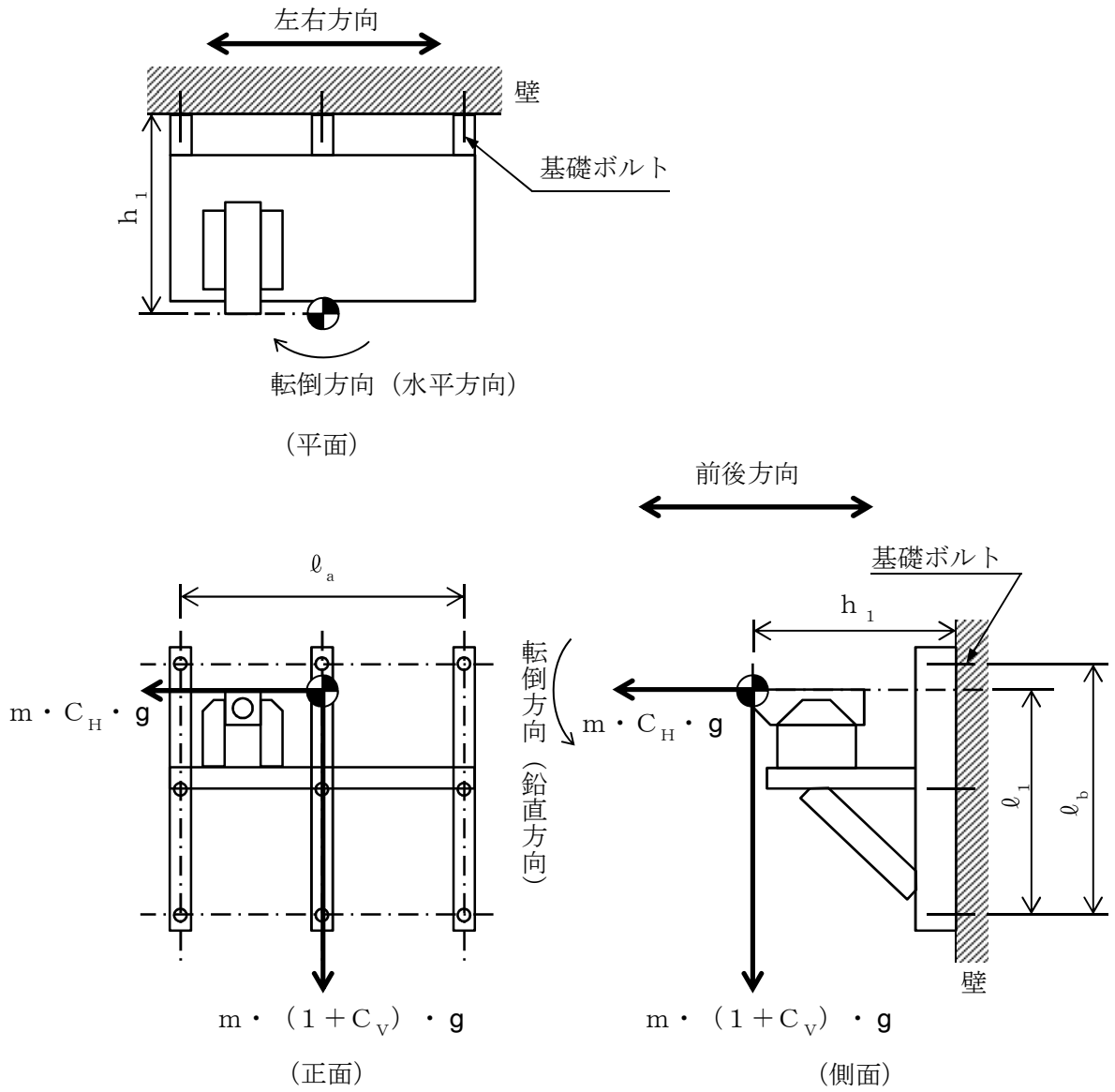
図5-4 熱感知カメラ 構造強度評価モデル
