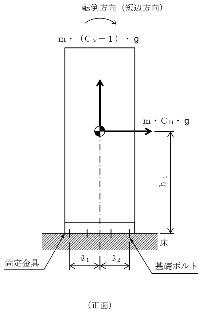
図5-6 火災受信機盤 短辺方向の構造強度評価モデル
