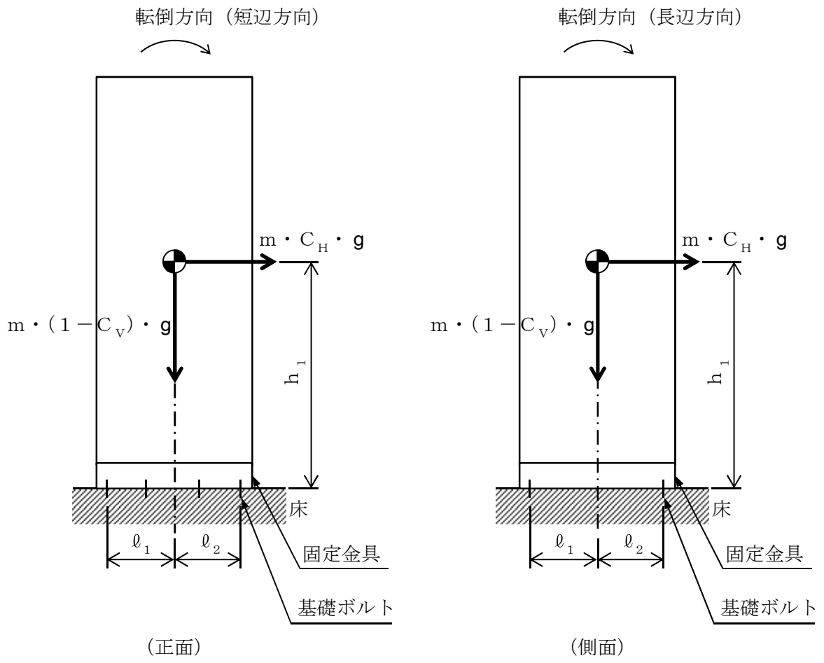
図5-8 制御監視盤 構造強度評価モデル
