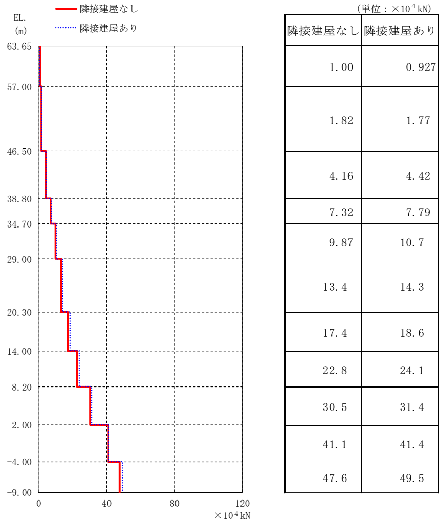
図 3-12 最大応答せん断力 ( , S_d - D 1 , EW 方向)
