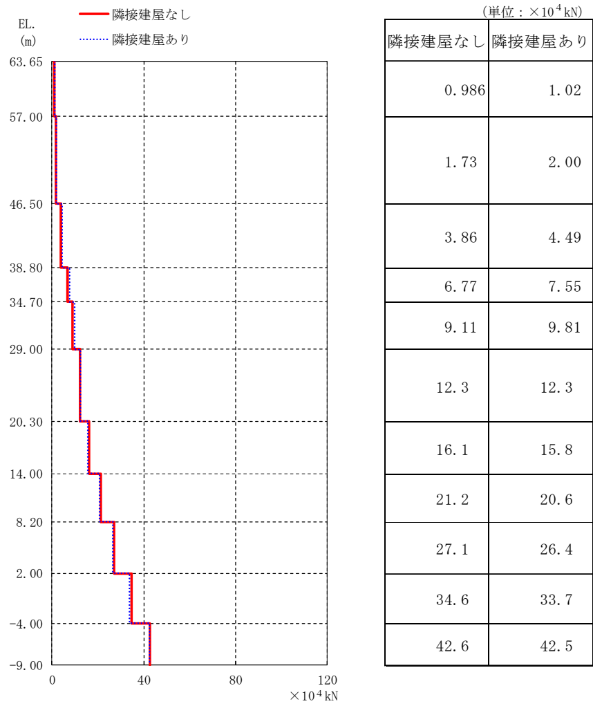
図 3-10 最大応答せん断力 ( S a -D 1, NS 方向)
