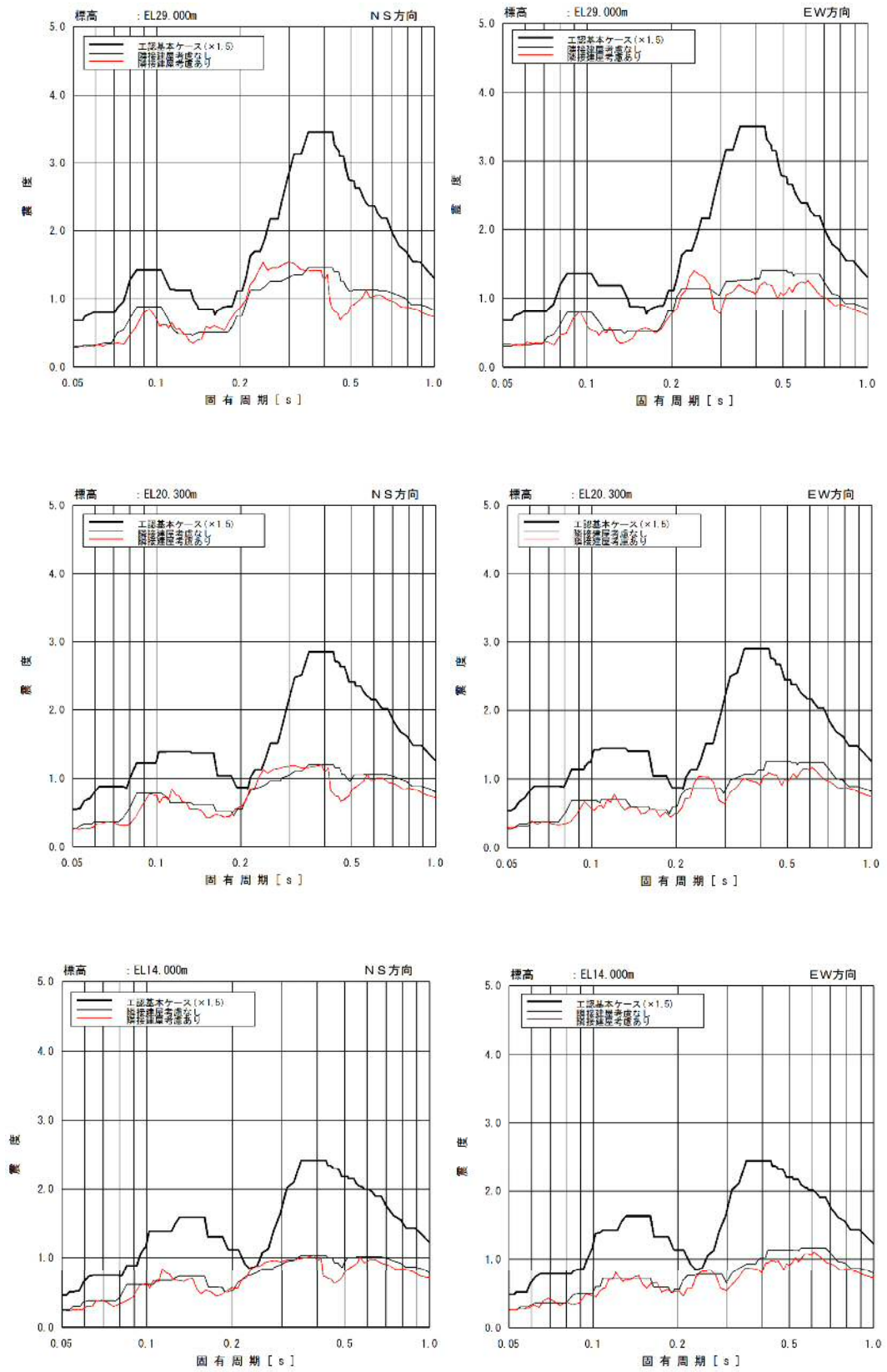
図3-13 (2/3) 床応答スペクトルの比較 (原子炉建屋 h=1.0%)
