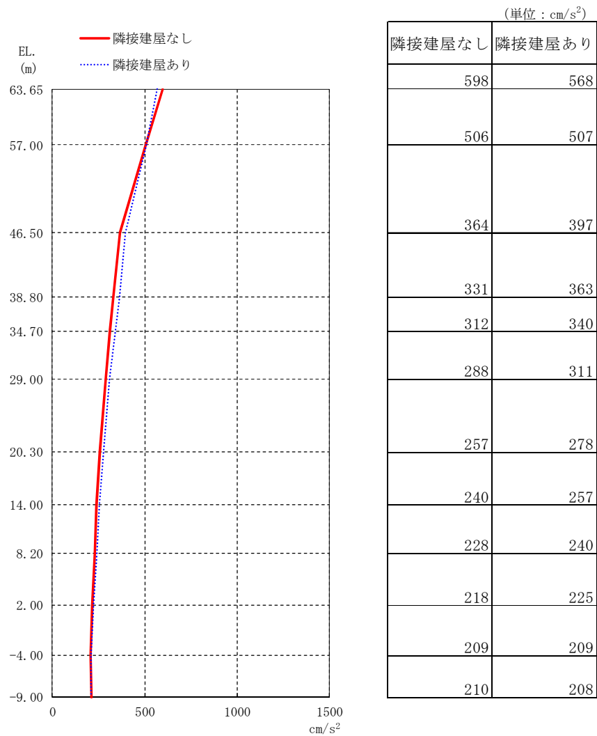
図 3-11 最大応答加速度 ( , S a -D1, EW 方向)
