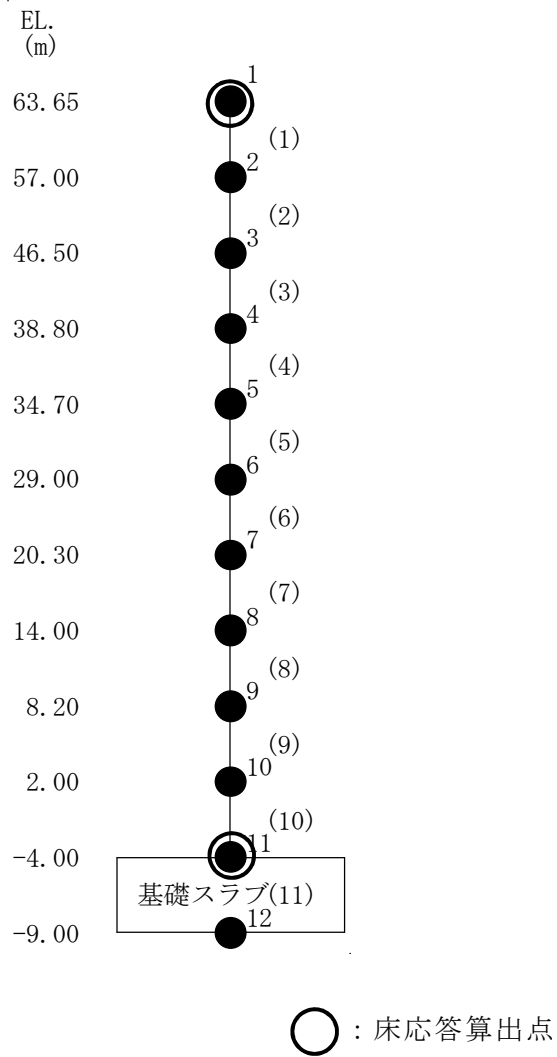
図 3-5 (R/B) の建屋モデル
