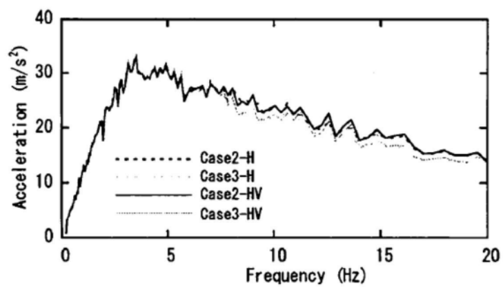
(a) 水平加速度応答スペクトル
