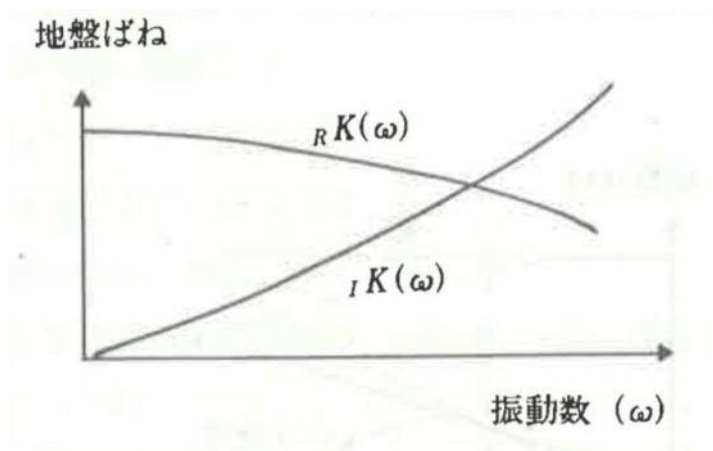
図 2-9 地盤ばねの近似
