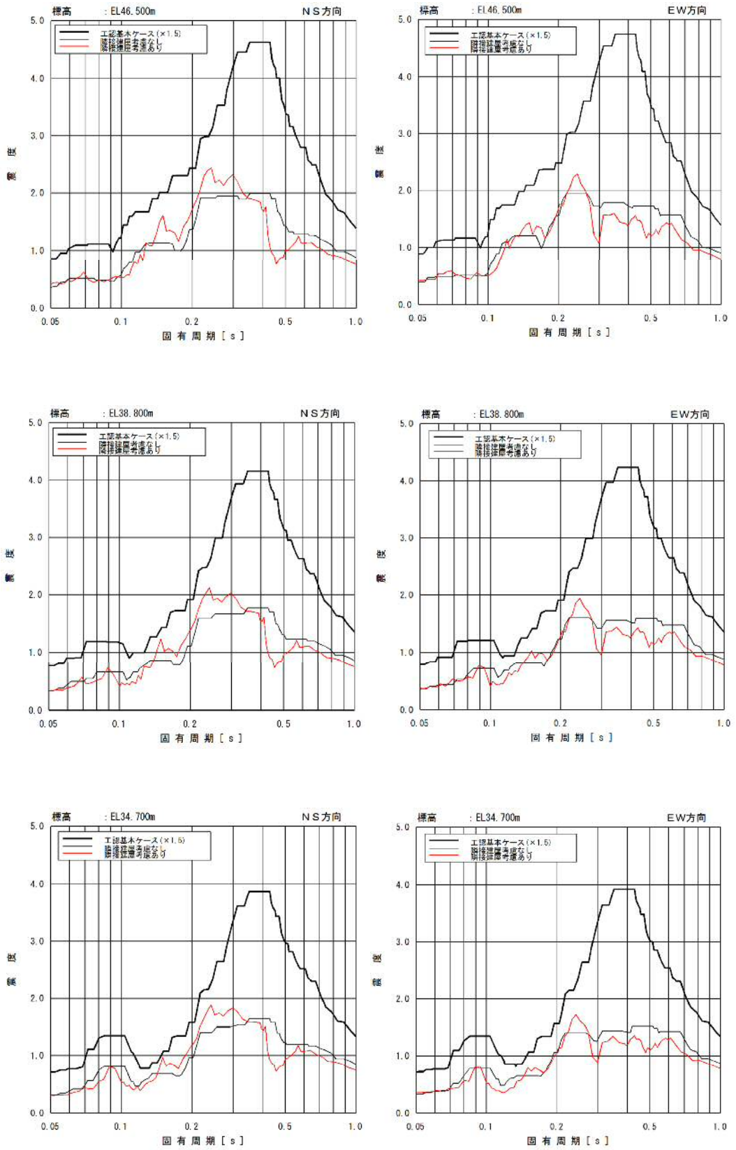
図3-13 (1/3) 床応答スペクトルの比較 (原子炉建屋 h=1.0\% )
