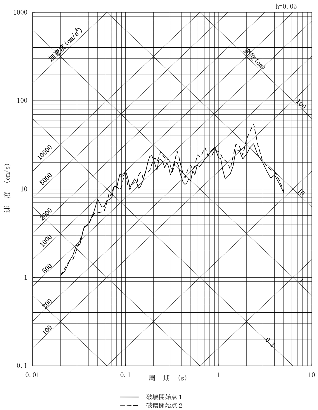
第6-30 図 (8) 茨城県南部の地震の断層モデルを用いた手法による地震動評価結果 (アスペリティ位置の不確かさを考慮, EW方向)
