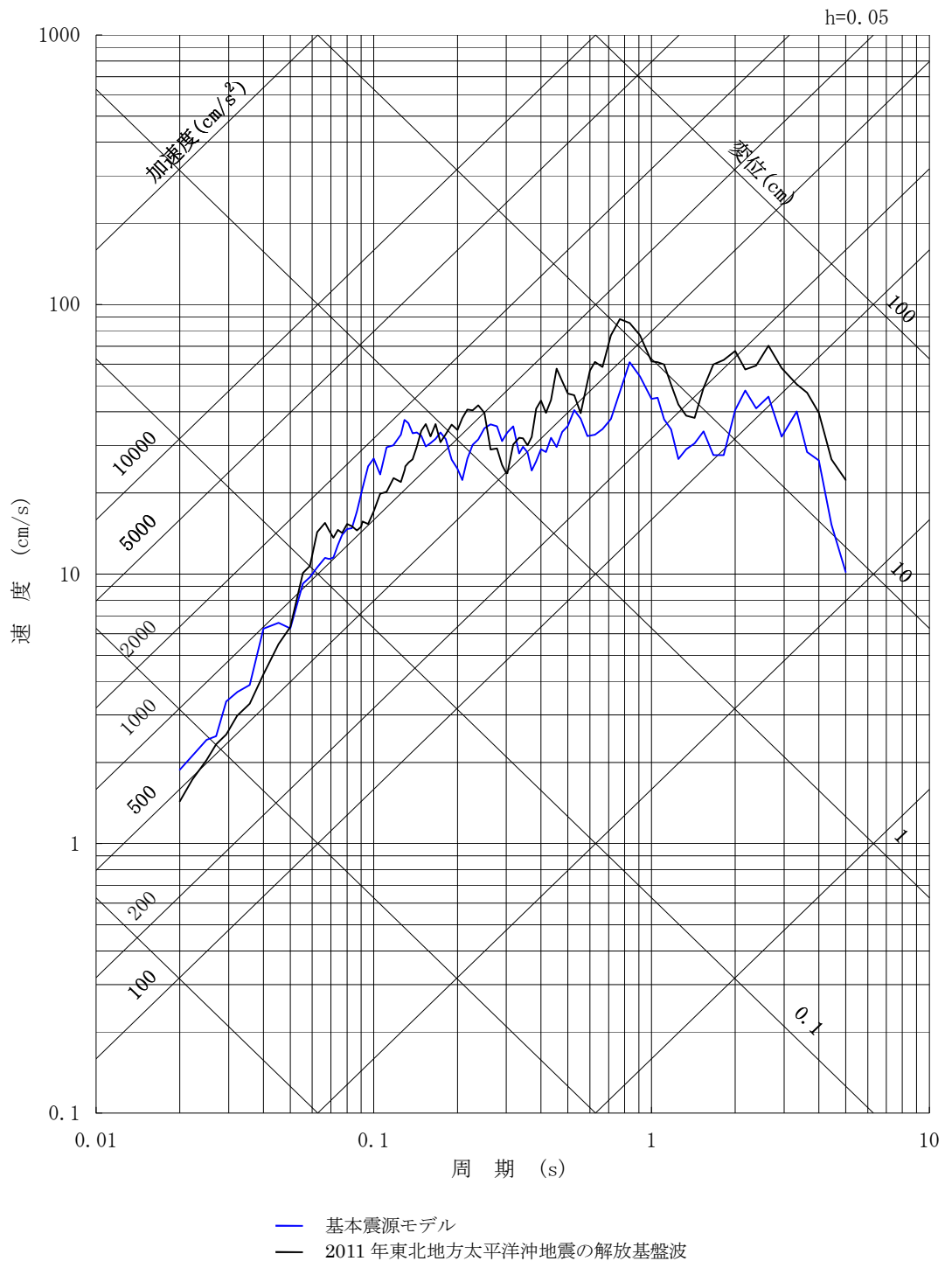
第6-18 図 (2) 2011年東北地方太平洋沖型地震の断層モデルを用いた手法による地震動評価果 (基本震源モデル) と 2011年東北地方太平洋沖地震の解放基盤波の比較 (EW 方向)
