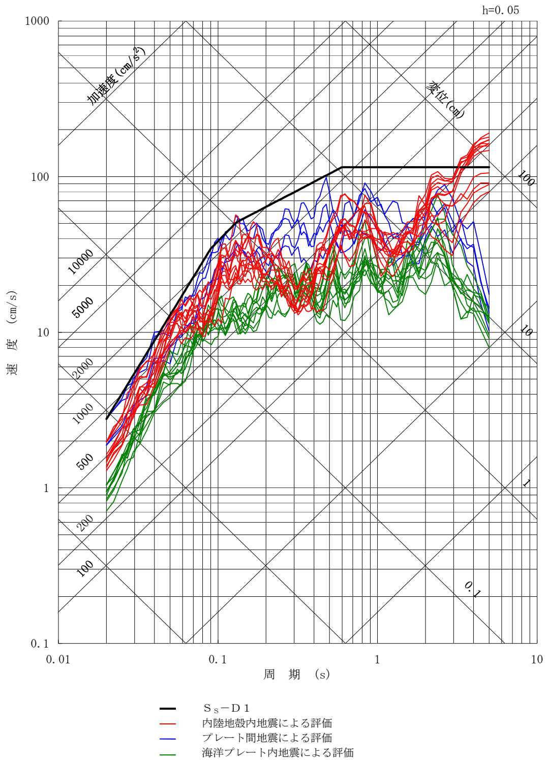
第6-34 図 (2) 基準地震動 S s -D 1 と断層モデルを用いた手法による地震動評価結果の比較 (E W方向)
