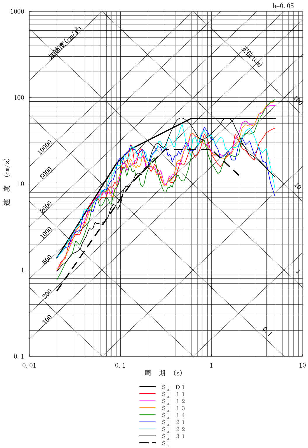
第8-5図(2) 弾性設計用地震動 S_d と基準地震動 S_1 の応答スペクトルの比較 (EW方向)
