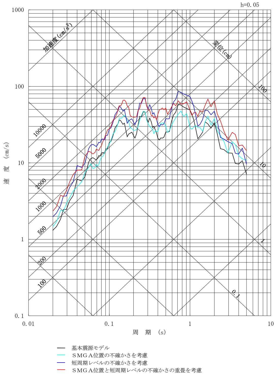
第6-17 図 (3) 2011年東北地方太平洋沖型地震の断層モデルを用いた手法による地震動評価結果 (基本震源モデル及び不確かさを考慮した各評価, UD方向)
