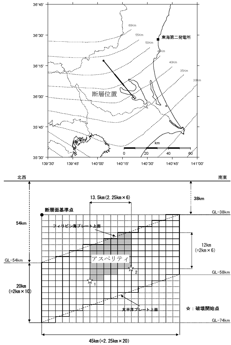
第 6-25 図 茨城県南部の地震の断層モデル (アスペリティ位置の不確かさを考慮)
