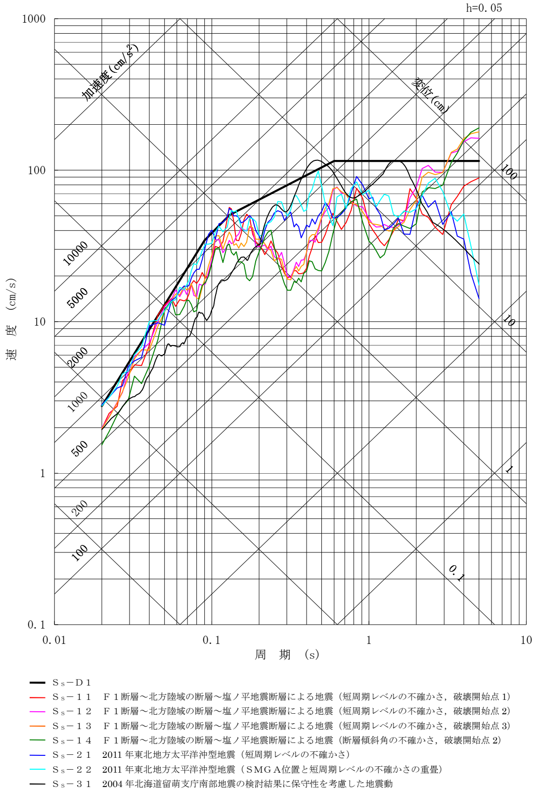
第6-41 図 (2) 基準地震動 S s の応答スペクトル (EW方向)
