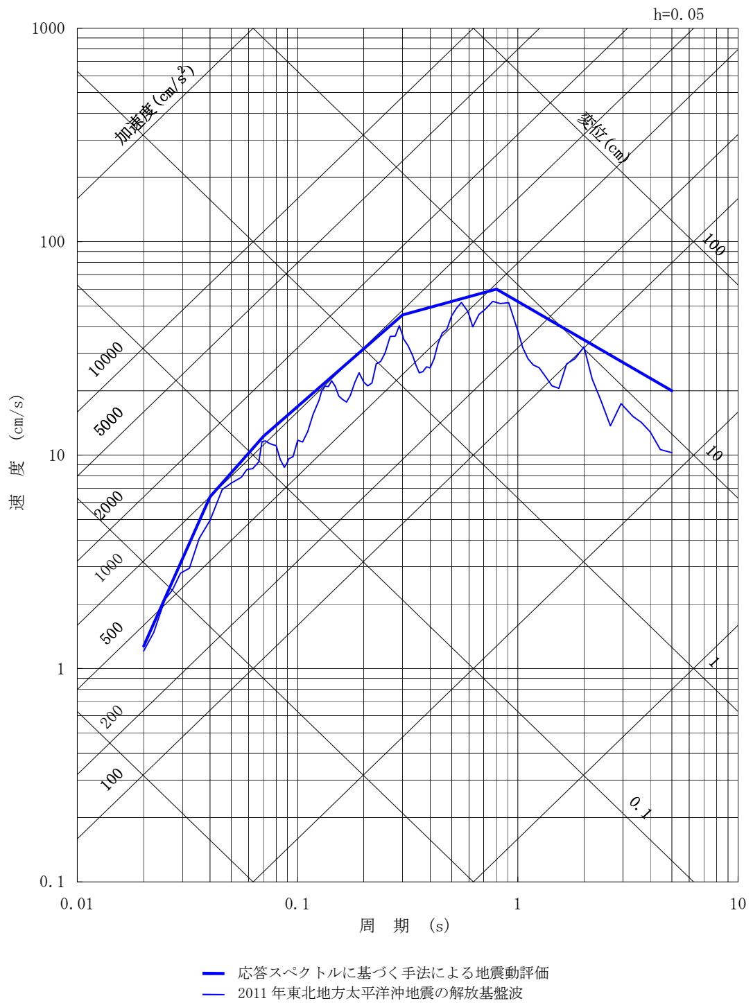
第6-15 図 (2) 2011年東北地方太平洋沖型地震の応答スペクトルに基づく手法による地震動評価結果と2011年東北地方太平洋沖地震の解放基盤波の比較 (鉛直方向)
