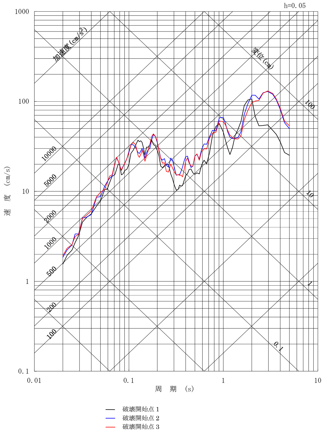
第6-9図(1) F1断層～北方陸域の断層～塩ノ平地震断層による地震の断層モデルを用いた手法による地震動評価結果(基本震源モデル, NS方向)
