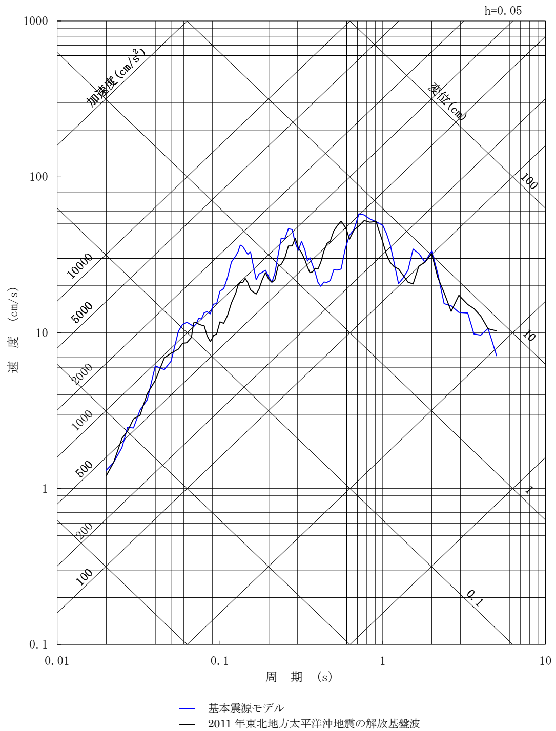
第6-18 図 (3) 2011年東北地方太平洋沖型地震の断層モデルを用いた手法による地震動評価果 (基本震源モデル) と 2011年東北地方太平洋沖地震の解放基盤波の比較 (UD 方向)
