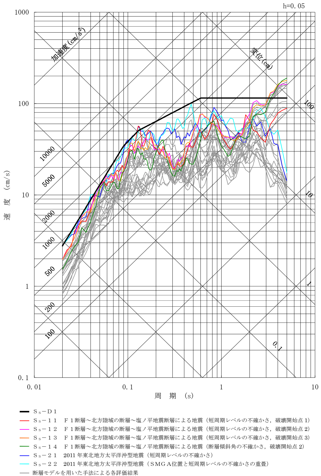
第 6-35 図 (2) 基準地震動 S s -D 1 と断層モデルを用いた手法による基準地震動 S s の比較 (E W 方向)
