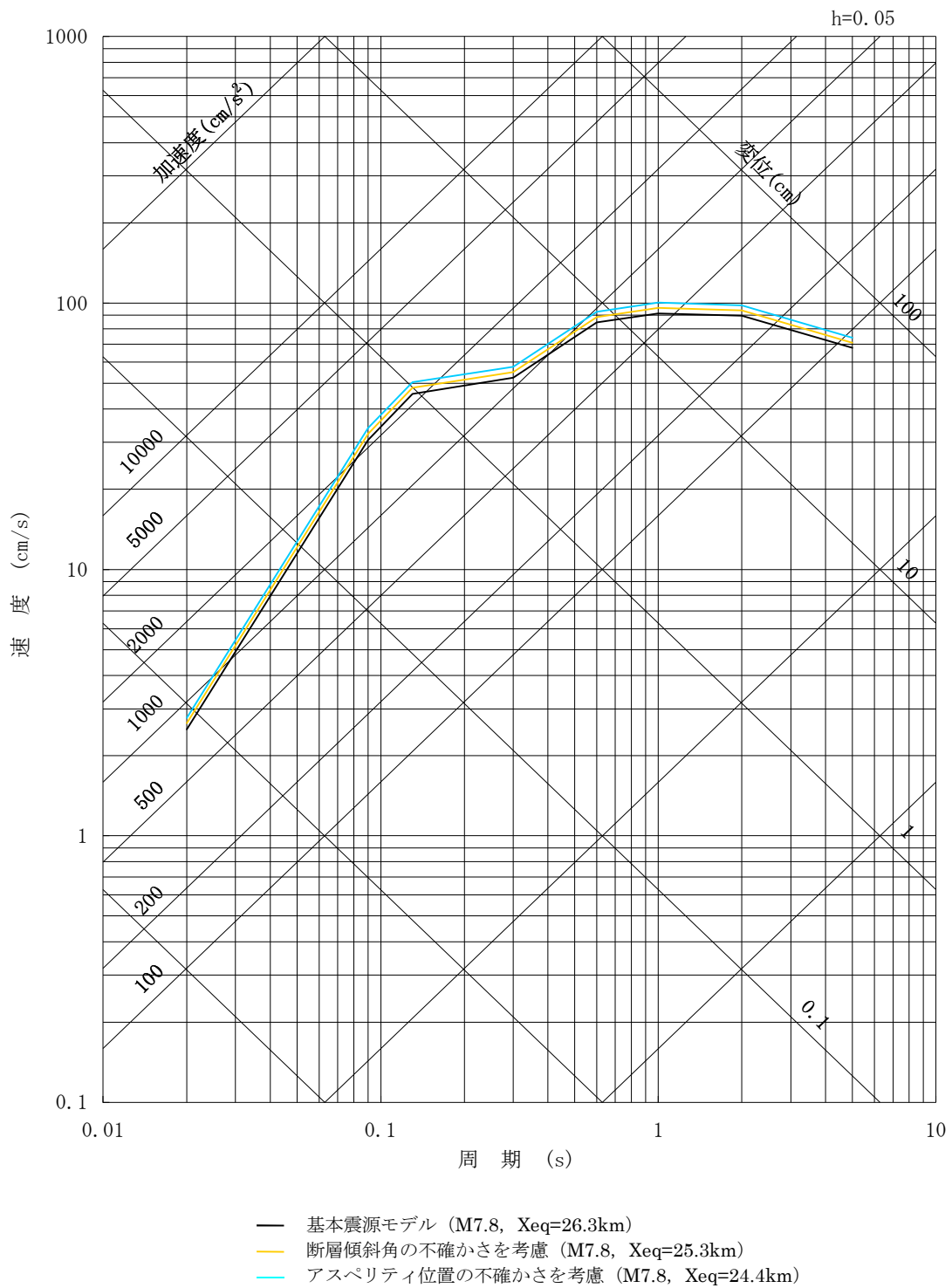
第6-7図(1) F1断層～北方陸域の断層～塩ノ平地震断層による地震の応答スペクトルに基づく手法による地震動評価結果(水平方向)
