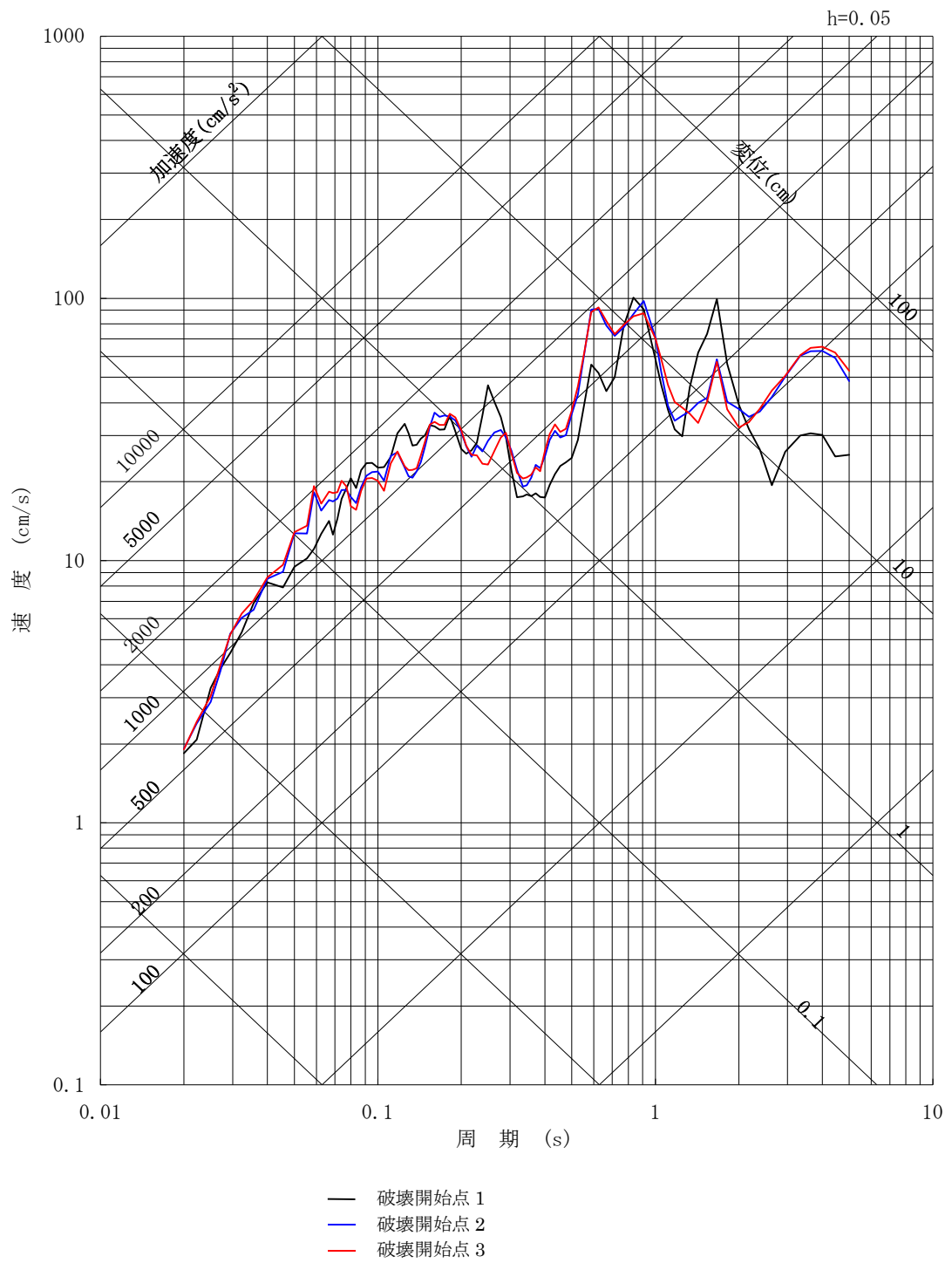
第6-9図(6) F1断層～北方陸域の断層～塩ノ平地震断層による地震の断層モデルを用いた手法による地震動評価結果(短周期レベルの不確かさを考慮, UD方向)
