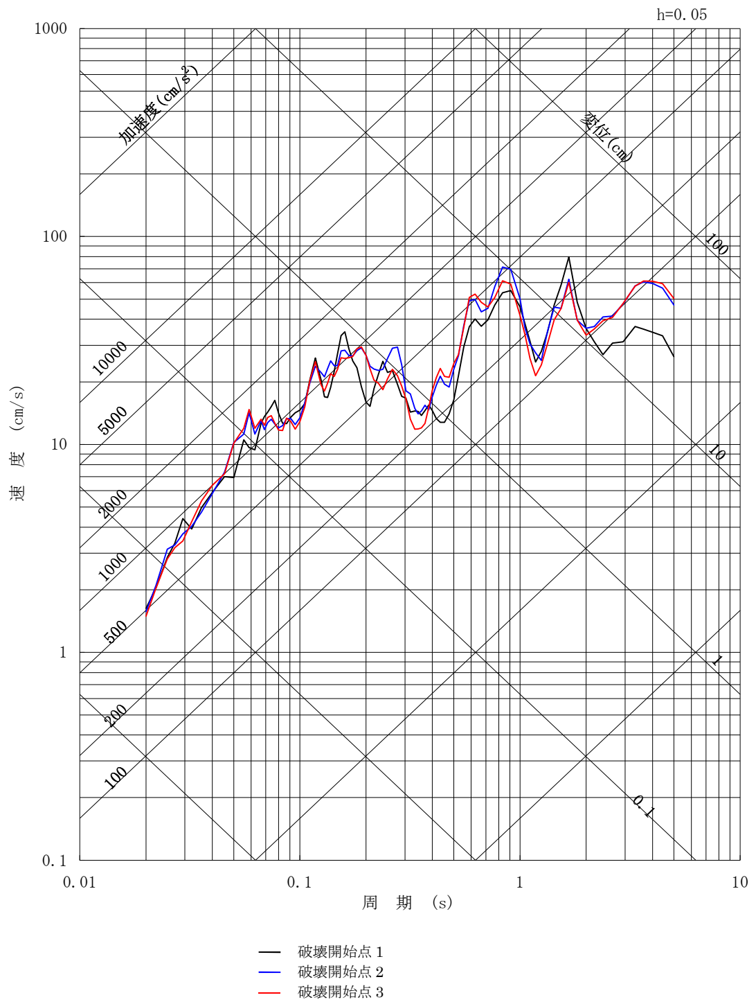
第6-9図 (12) F1断層～北方陸域の断層～塩ノ平地震断層による地震の断層モデルを用いた手法による地震動評価結果 (アスペリティ位置の不確かさを考慮, UD方向)
