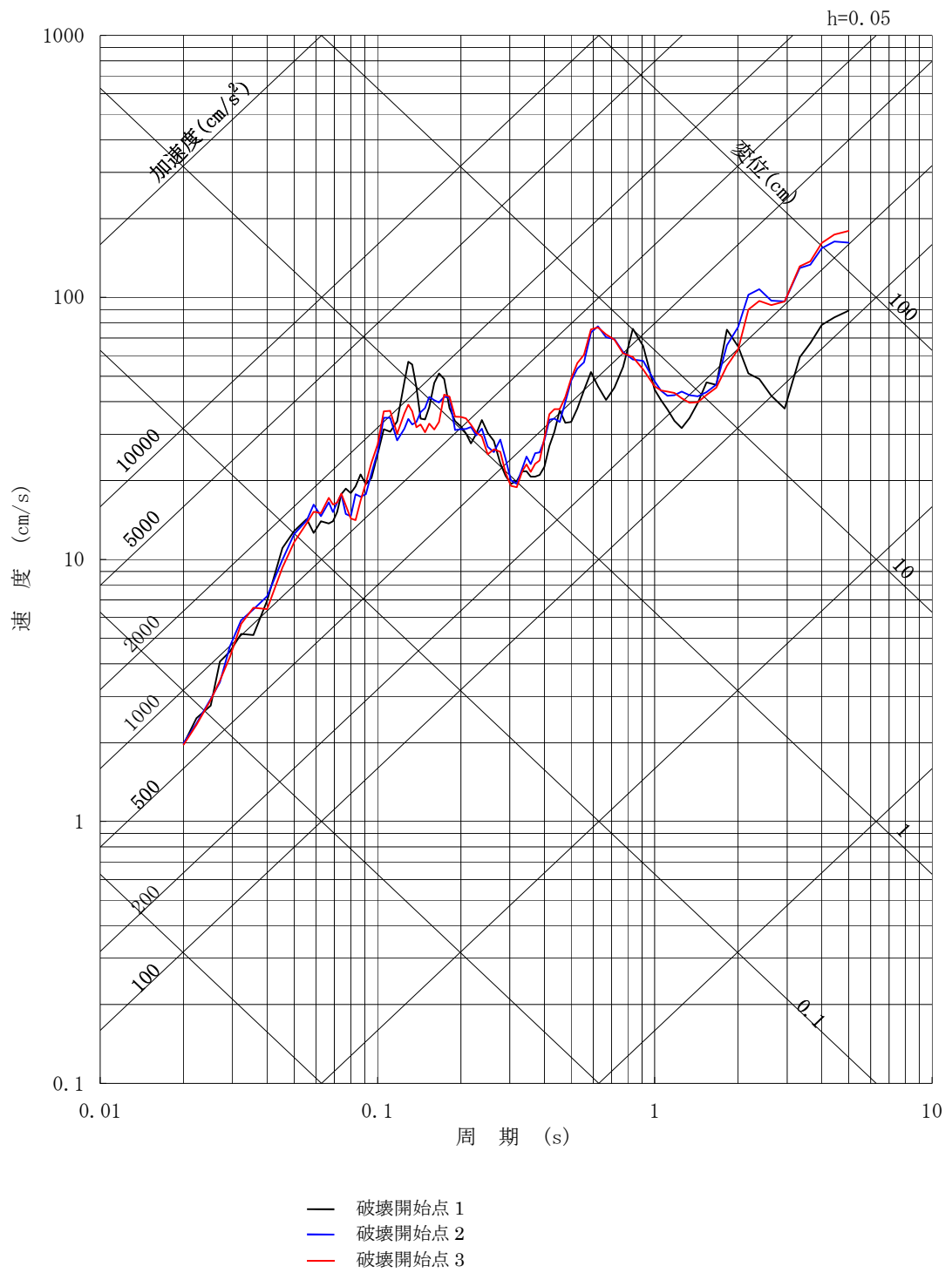
第6-9図 (5) F1断層～北方陸域の断層～塩ノ平地震断層による地震の断層モデルを用いた手法による地震動評価結果 (短周期レベルの不確かさを考慮, EW方向)
