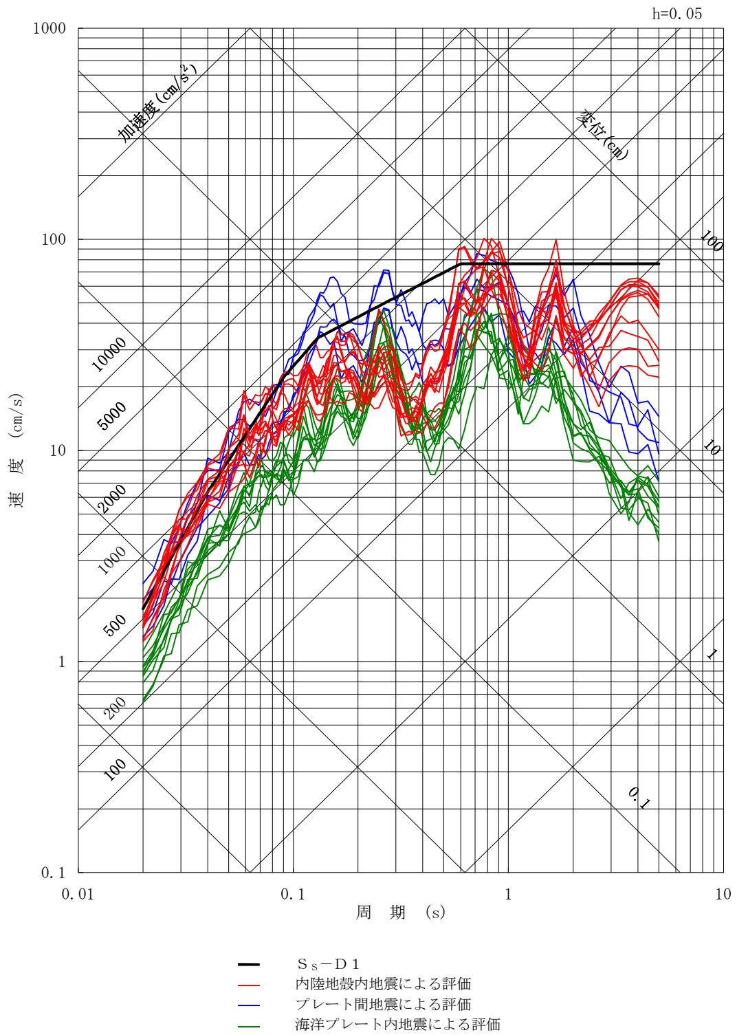
第6-34 図 (3) 基準地震動 S s -D 1 と断層モデルを用いた手法による地震動評価結果の比較 (UD方向)
