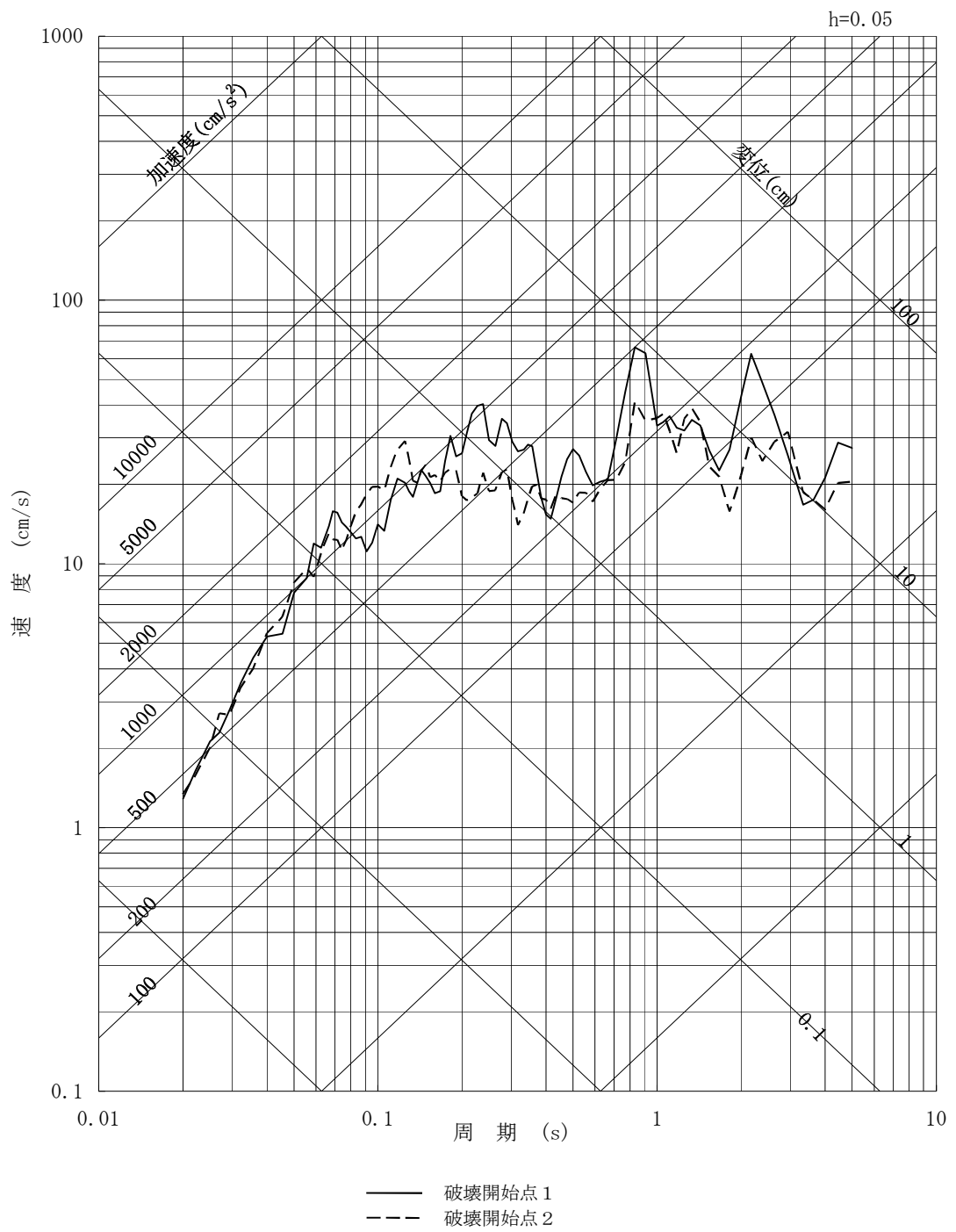
第6-30 図 (10) 茨城県南部の地震の断層モデルを用いた手法による地震動評価結果 (応力降下量の不確かさを考慮, NS方向)
