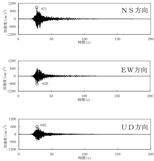
第6-39 図 (2) 基準地震動 S s -1-2 の時刻歴波形
