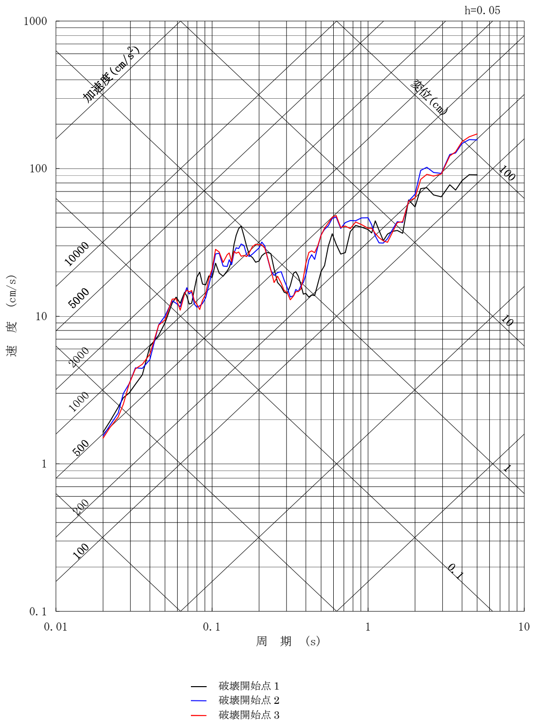
第6-9図 (11) F1断層～北方陸域の断層～塩ノ平地震断層による地震の断層モデルを用いた手法による地震動評価結果 (アスペリティ位置の不確かさを考慮, EW方向)
