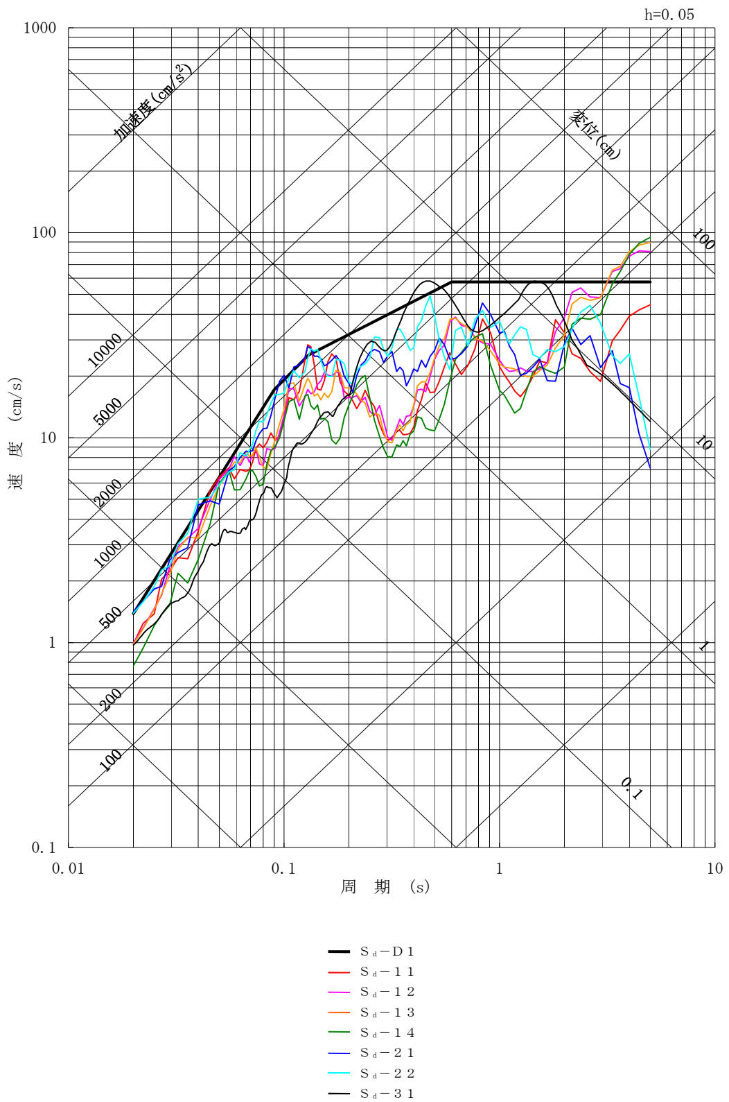
第8-1図(2) 弾性設計用地震動S d の応答スペクトル(EW方向)
