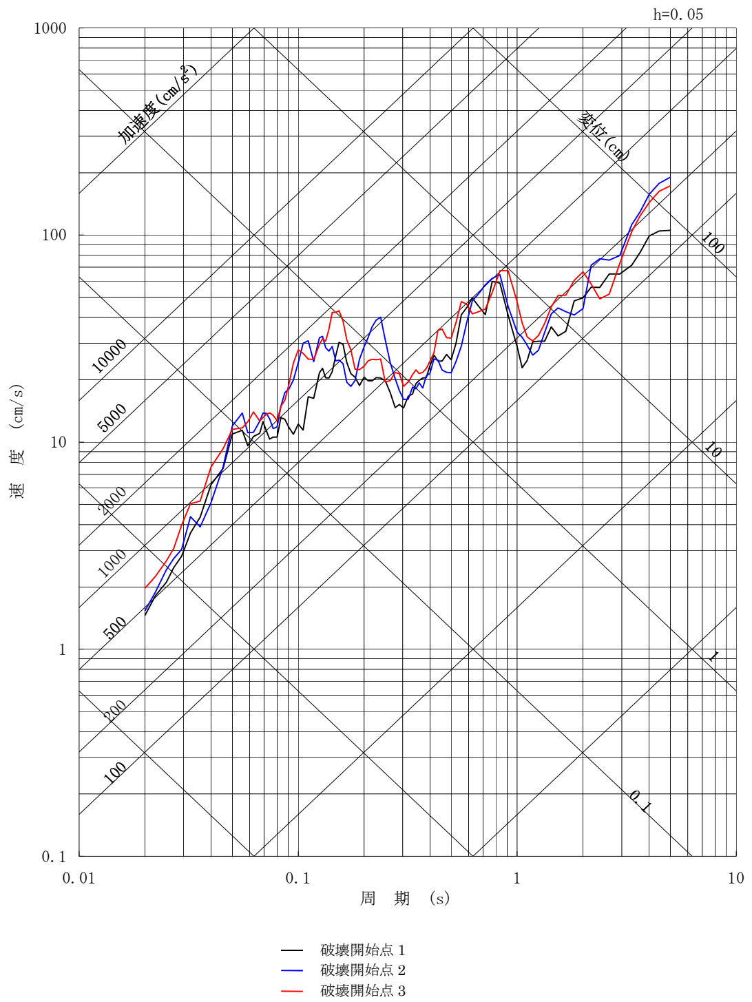
第6-9図(8) F1断層～北方陸域の断層～塩ノ平地震断層による地震の断層モデルを用いた手法による地震動評価結果(断層傾斜角の不確かさを考慮, EW方向)
