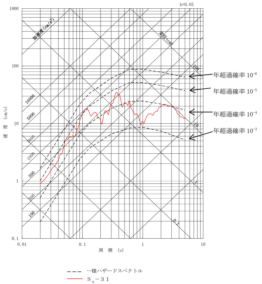
第7-18 図 (2) 内陸地殻内地震の領域震源モデルによる一様ハザードスペクトルと基準地震動 S s -31 の応答スペクトルの比較 (鉛直方向)
