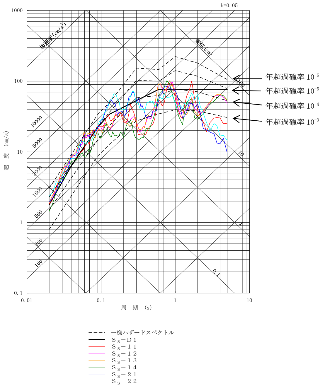
第7-17 図 (2) 一様ハザードスペクトルと基準地震動 S_s-D1 , S_s-11 \sim S_s-22 の応答スペクトルの比較 (鉛直方向)
