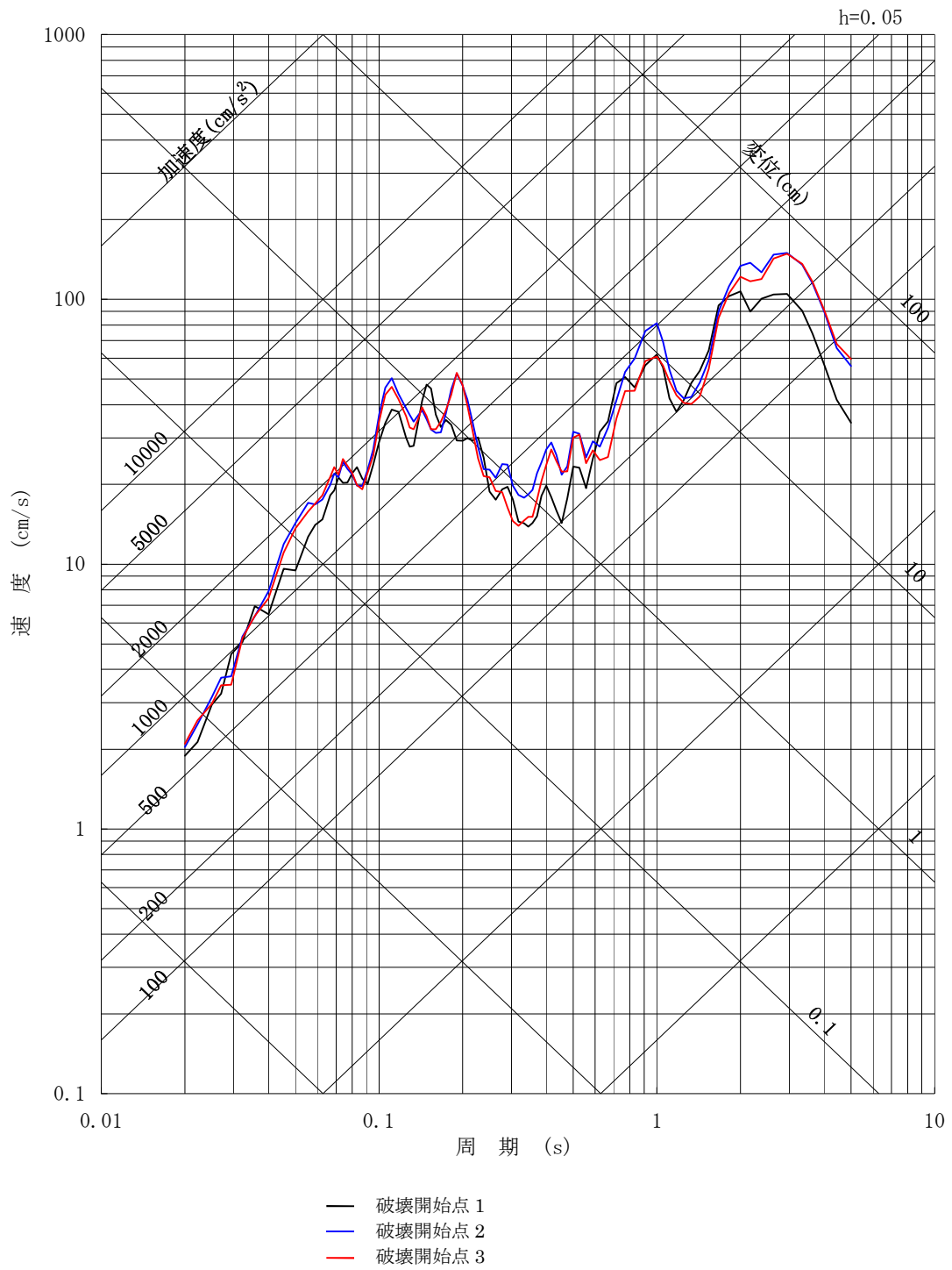
第 6-9 図 (10) F 1 断層～北方陸域の断層～塩ノ平地震断層による地震の断層モデルを用いた手法による地震動評価結果 (アスペリティ位置の不確かさを考慮, NS 方向)
