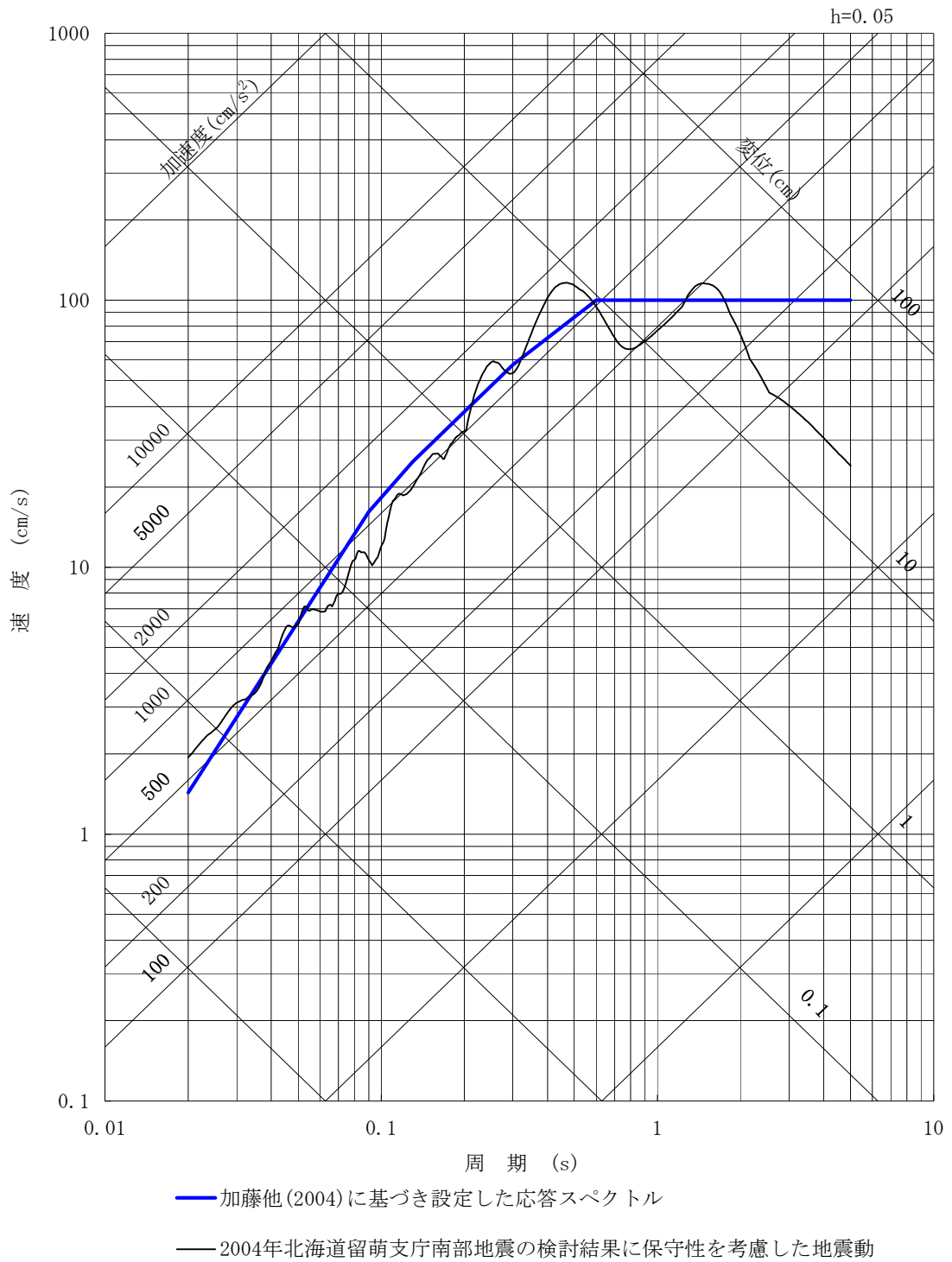
第6-32 図 (1) 震源を特定せず策定する地震動の応答スペクトル (水平方向)
