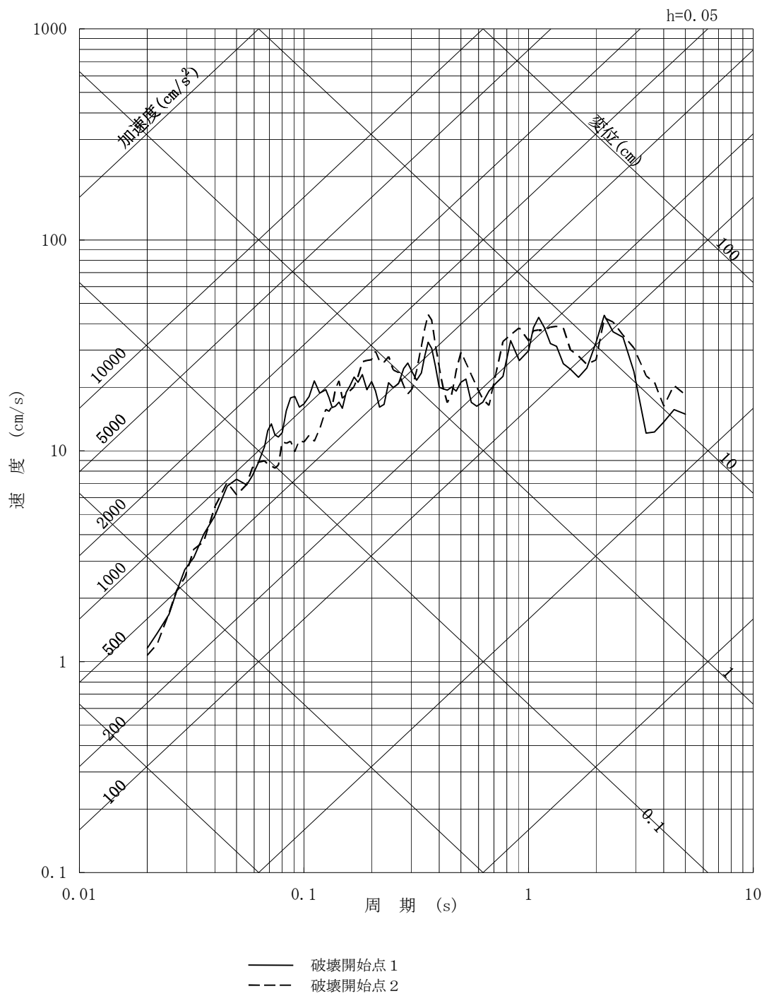
第6-30 図 (1) 茨城県南部の地震の断層モデルを用いた手法による地震動評価結果 (基本震源モデル, NS方向)
