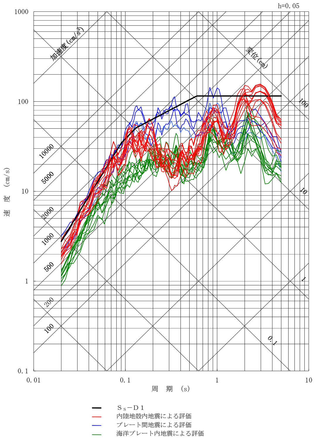
第6-34 図 (1) 基準地震動 S s -D 1 と断層モデルを用いた手法による地震動評価結果の比較 (NS方向)
