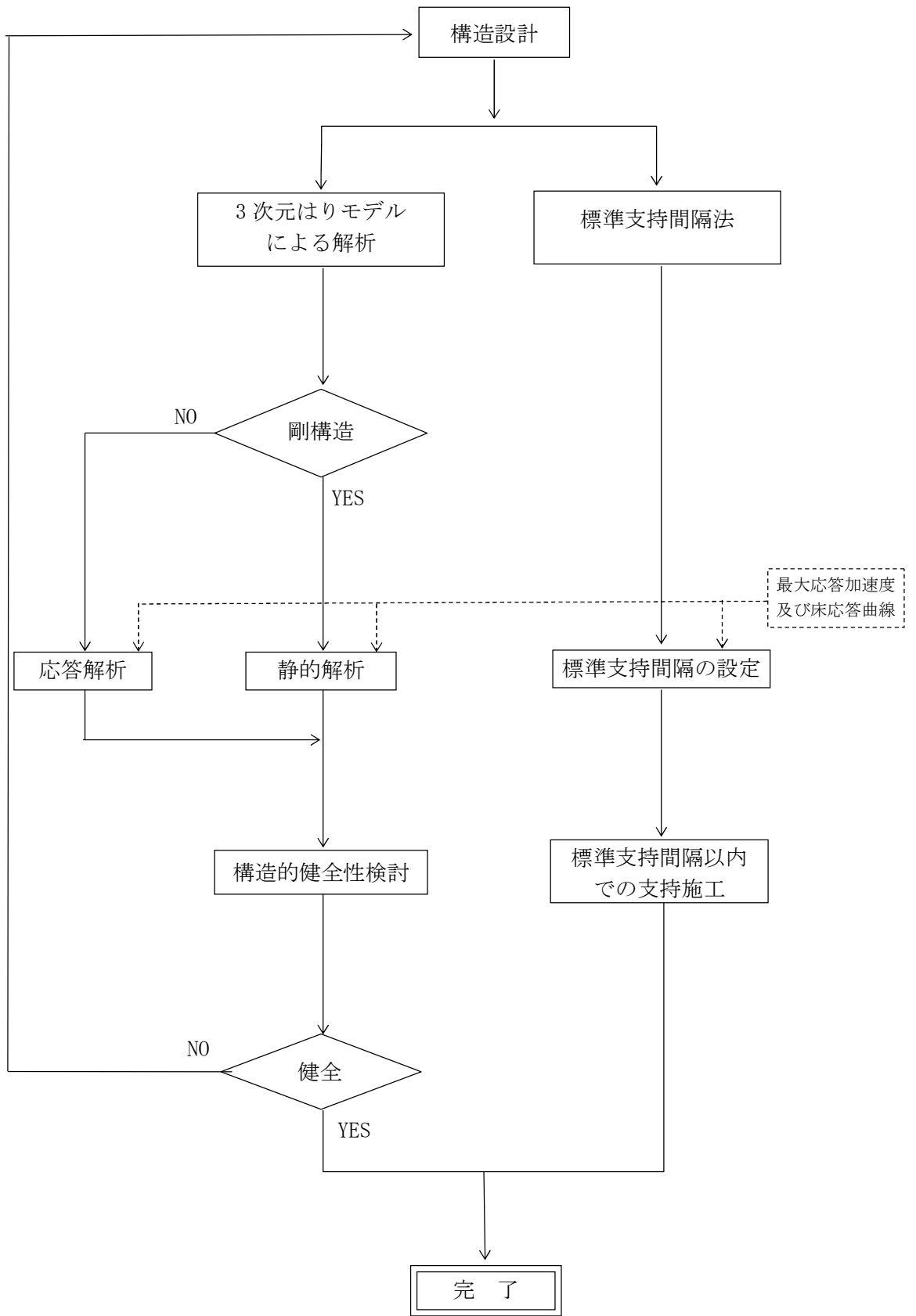
図 3-4 電路類の耐震設計フローチャート
