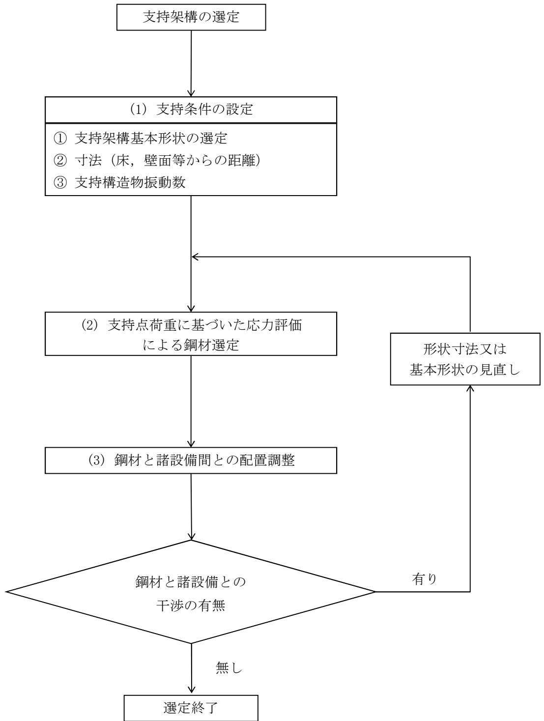
図4-4 支持架構の設計フロー
