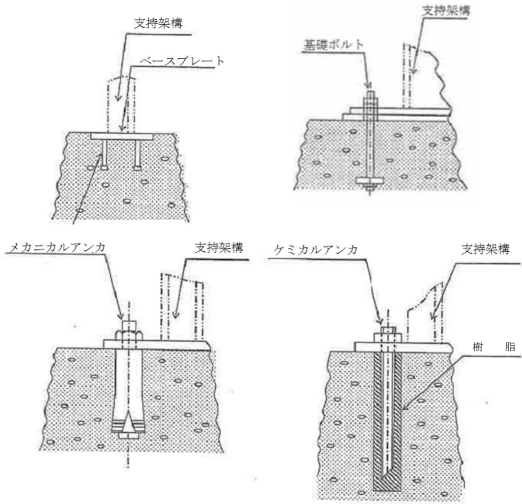
図4-6 埋込金物の例
