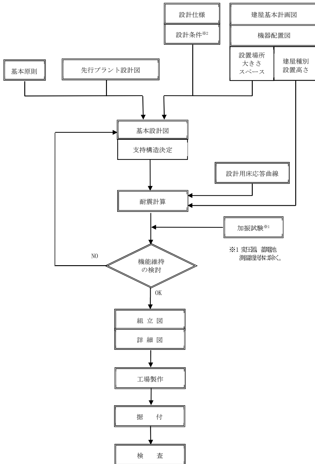
図3-1 電気計測制御装置の支持構造物設計フロー
