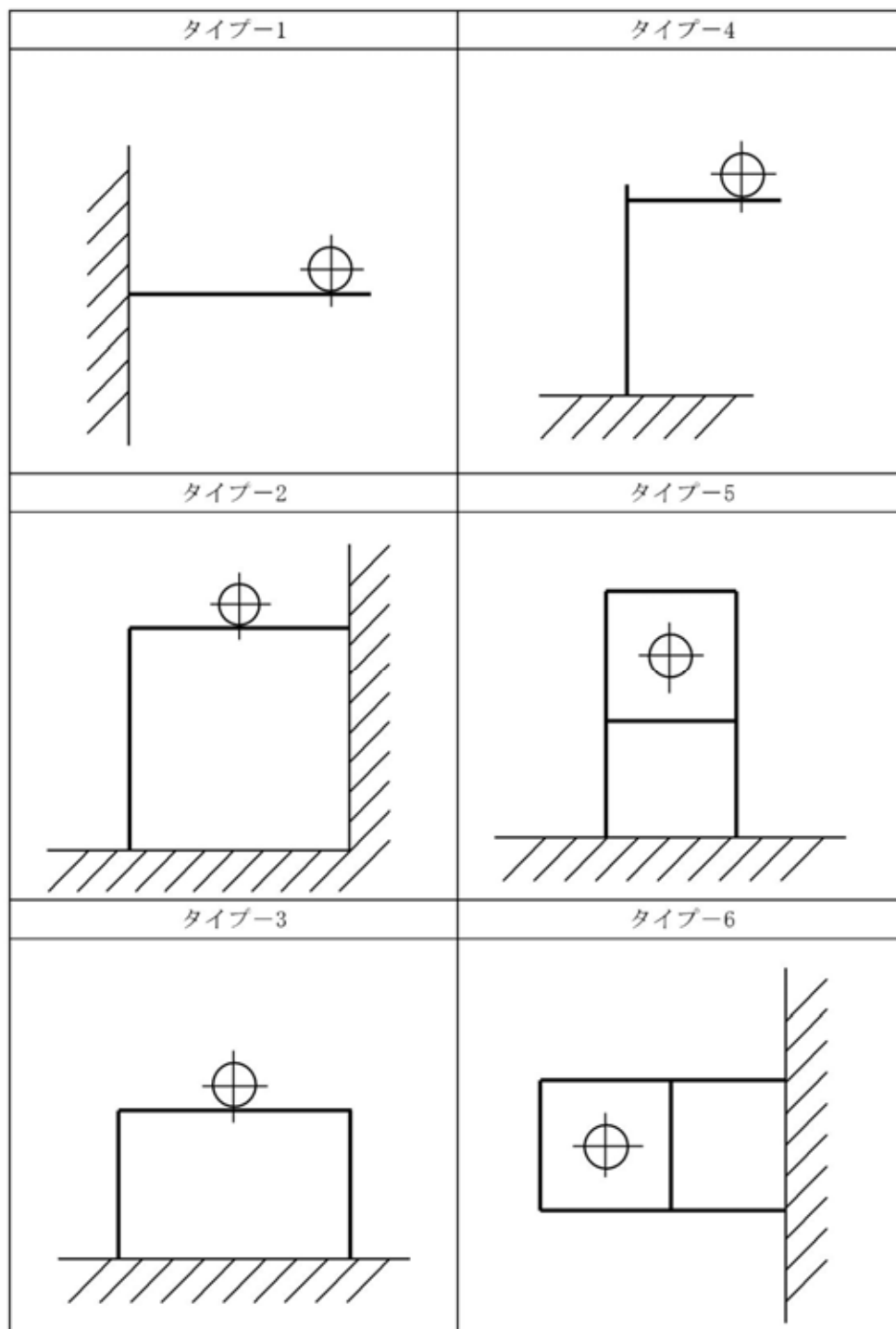
図4-3 支持架構の基本形状例
