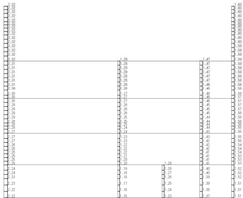
To2_PVB-E#_DG-Non-L_Ss-31+ Maximum Vertical Acceleration → 構造スケール 0 5 (m) → 応答値スケール 0 10 (m/sec 2 )
