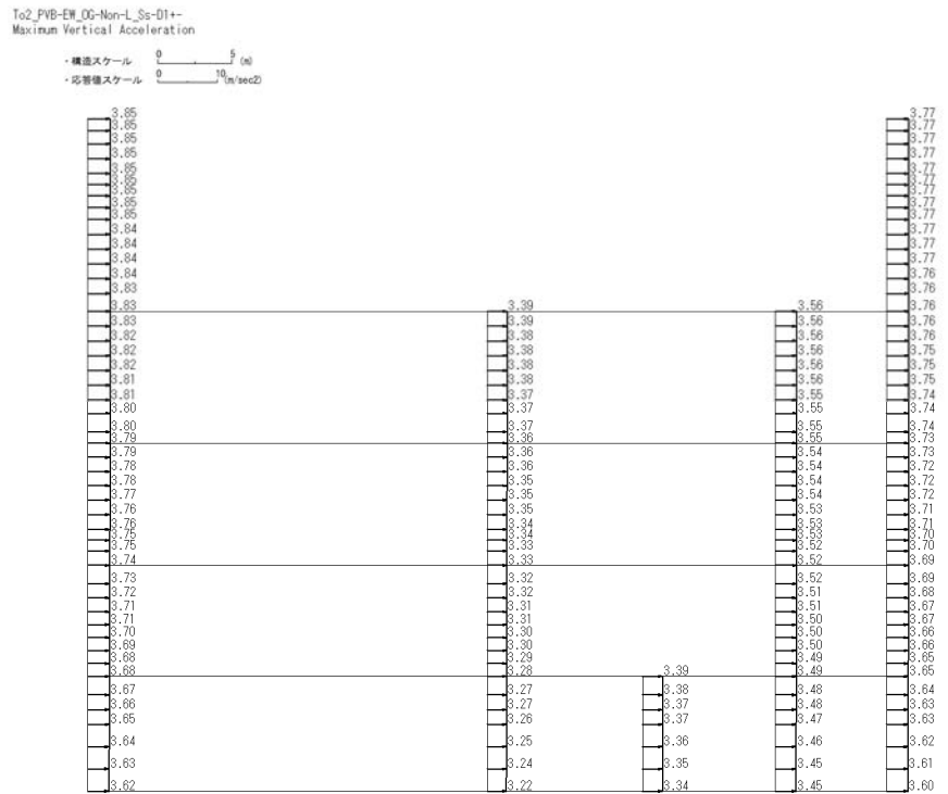
図 4-2 ⑤原地盤において非液状化の条件を仮定した解析ケース 最大加速度分布図 (1/10)
