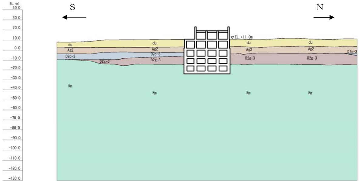
図 3-2 電源装置置場の評価対象断面図（南北方向断面）
