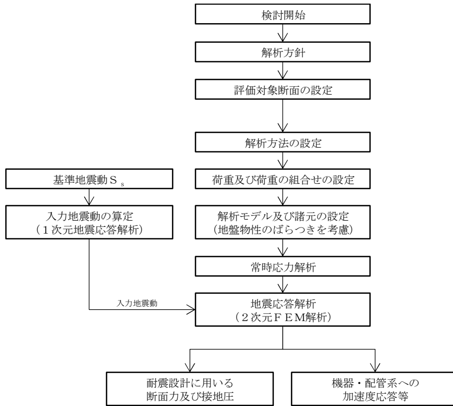
図 2-4 電源装置置場の地震応答解析フロー
