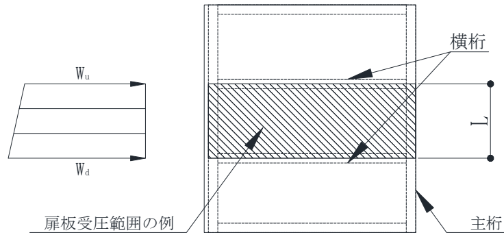
図3-2 扉板に生じる荷重の例
