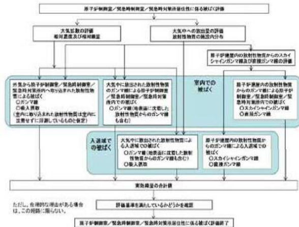
図3 原子炉制御室/緊急時対策所/緊急時対策所の居住性に係る被ばく評価手順
