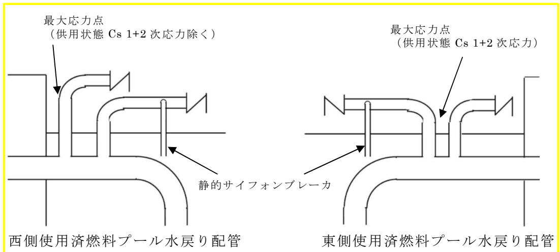
第7図 最大応力点位置
