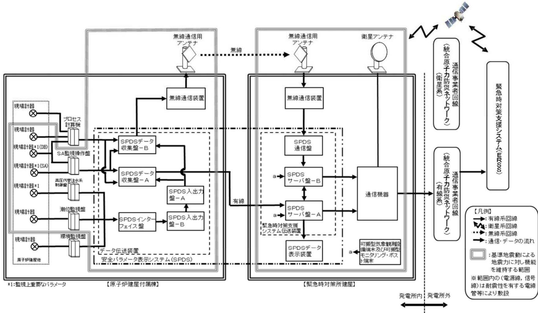
図3 安全パラメータ表示システム (SPDS) 及びデータ伝送設備の概略構成図
