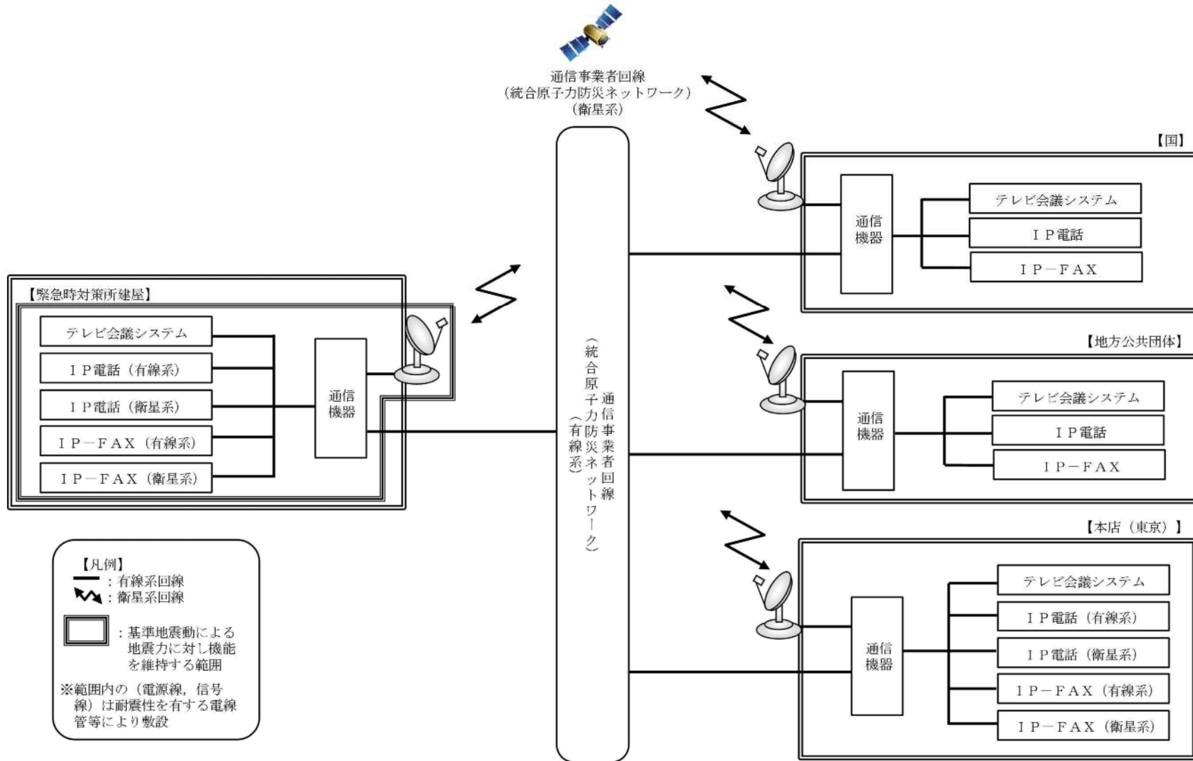
図4 統合原子力防災ネットワークに接続する通信連絡設備(テレビ会議システム, IP電話及びIP-FAX)の概略構成図
