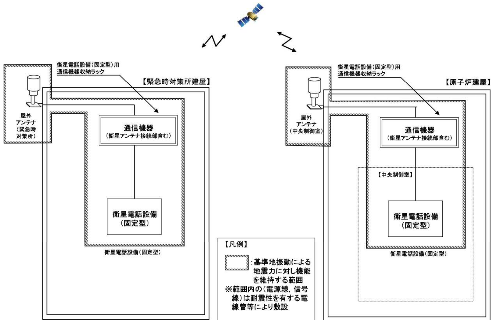
図2 衛星電話設備 (固定型) 概略構成図
