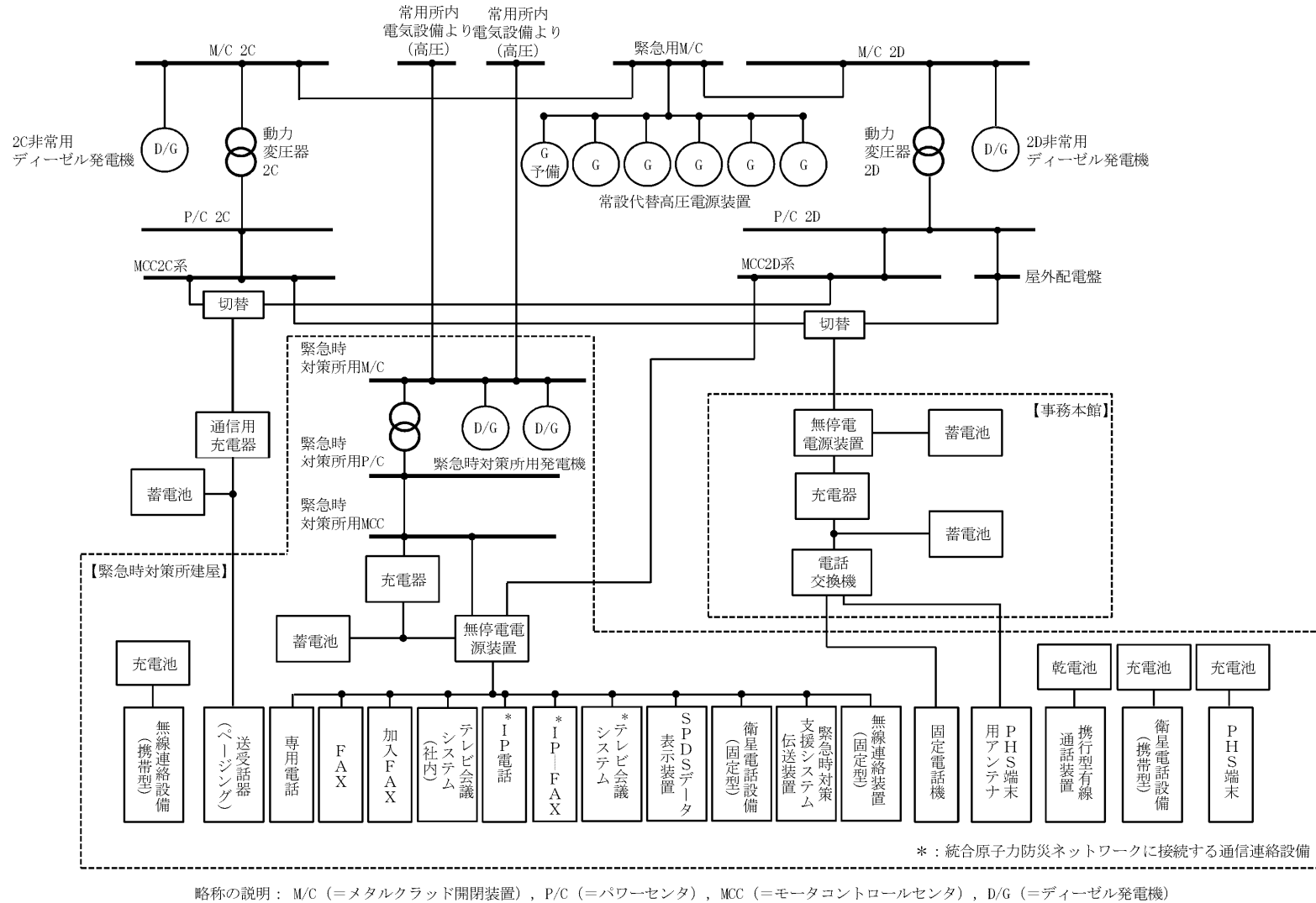
図1 通信連絡設備の電源概略構成図 (2/2)
