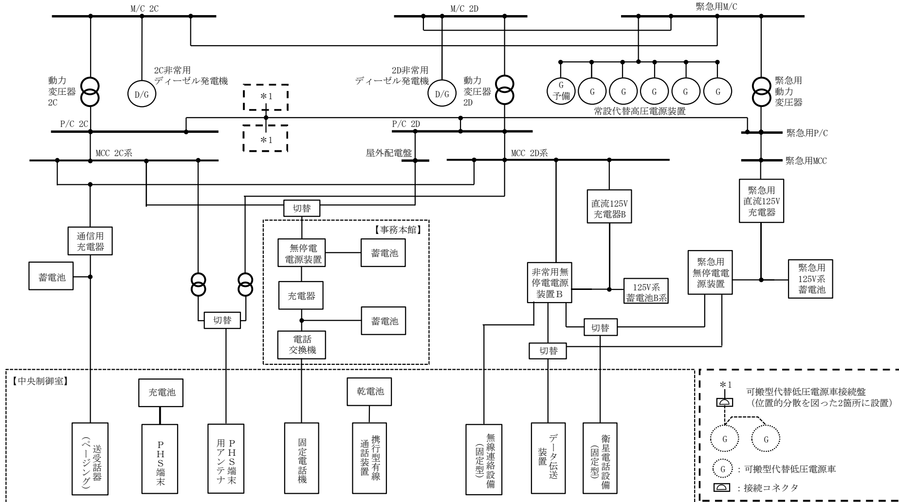
図1 通信連絡設備の電源概略構成図 (1/2)
