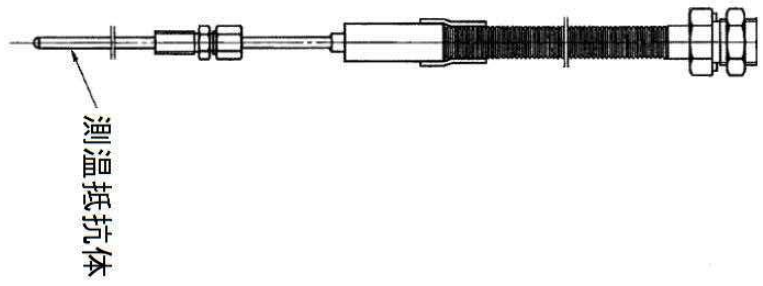
図4-23 温度検出器の構造概要
