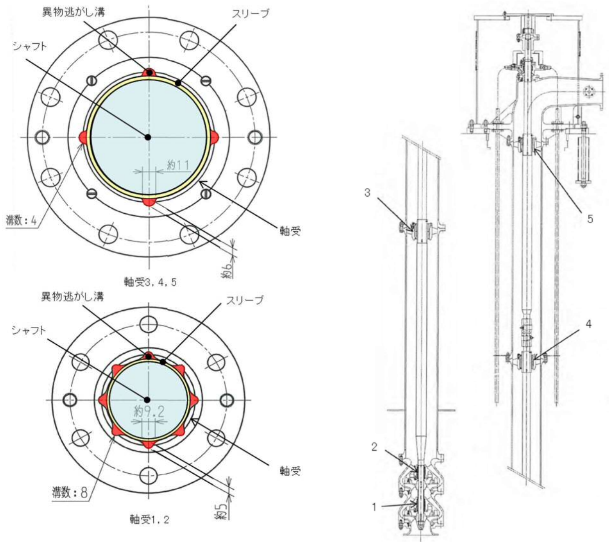
図 1-4 非常用ディーゼル発電機（高圧炉心スプレイ系ディーゼル発電機を含む。）用海水ポンプ 軸受部詳細
