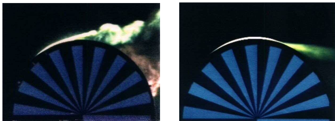
図 5-4 可視化した円柱まわりの流れ (21)
