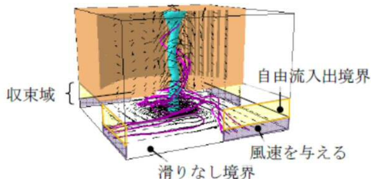
図2-5 LES計算領域内での竜巻状の渦の作成状況
