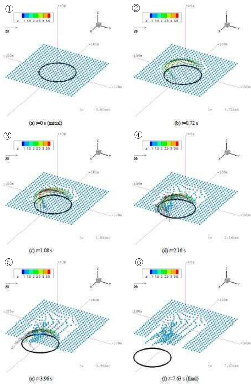
図 5-15 竜巻によるトラックの飛散イメージ (23) (表 6-5 (後述) の条件による)
