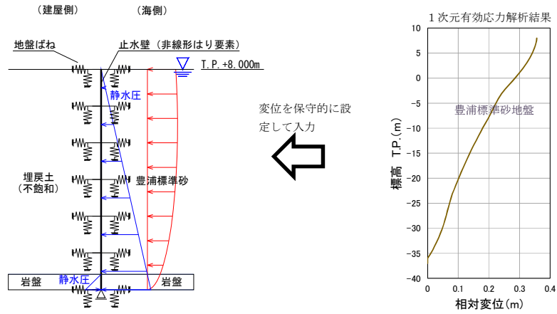
図 2.1.1-5 応答変位法解析モデル図
