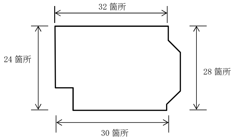
図 2.1.1-8 止水壁の施工継目箇所図
