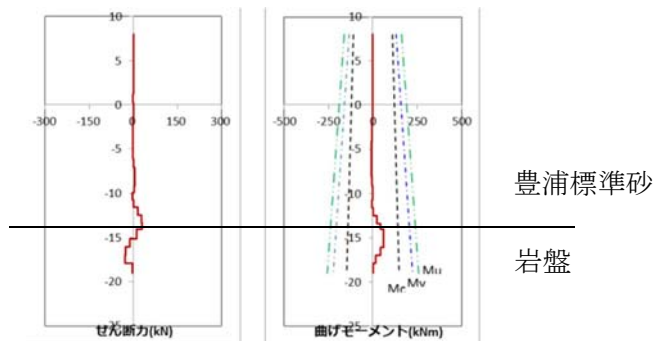
図 2. 1. 1-6 (1) 断面力図 (岩盤が浅い位置)
