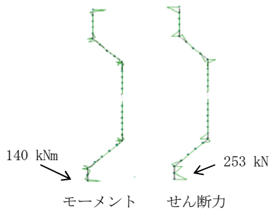
図 2.1.1-13 評価結果図 (断面力図)
