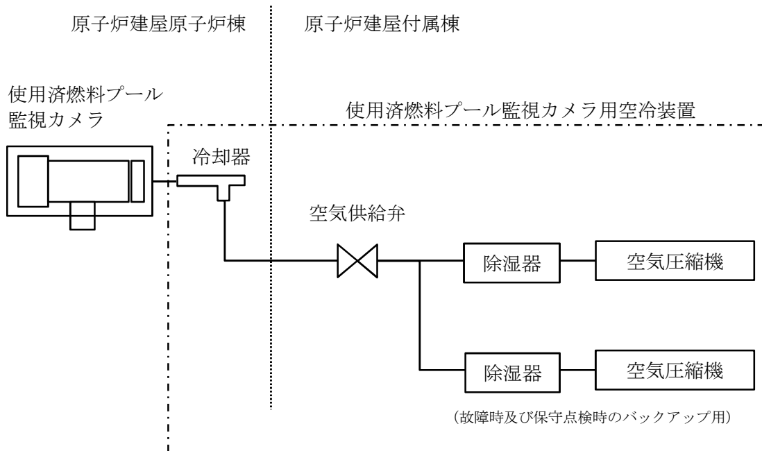
図 2. 2. 1-2 使用済燃料プール監視カメラ用空冷装置の空気供給概略図
