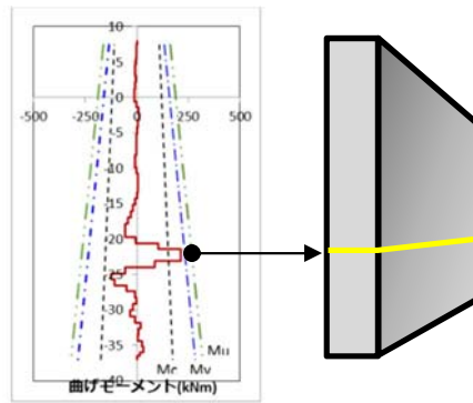
図 2.1.1-9 水平方向ひび割れ仮定位置図
