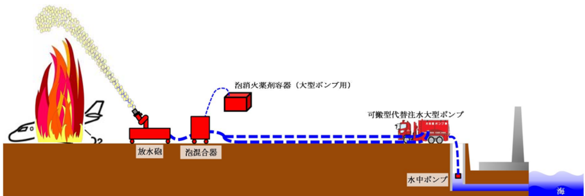
図 2.5.2-1 航空機燃料火災への泡消火 系統概要図
