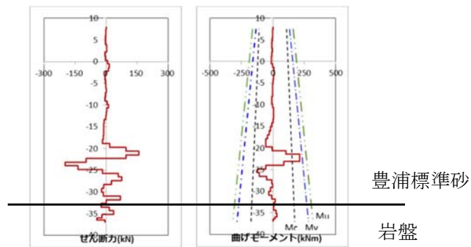
図 2. 1. 1-6 (2) 断面力図 (岩盤が深い位置)
