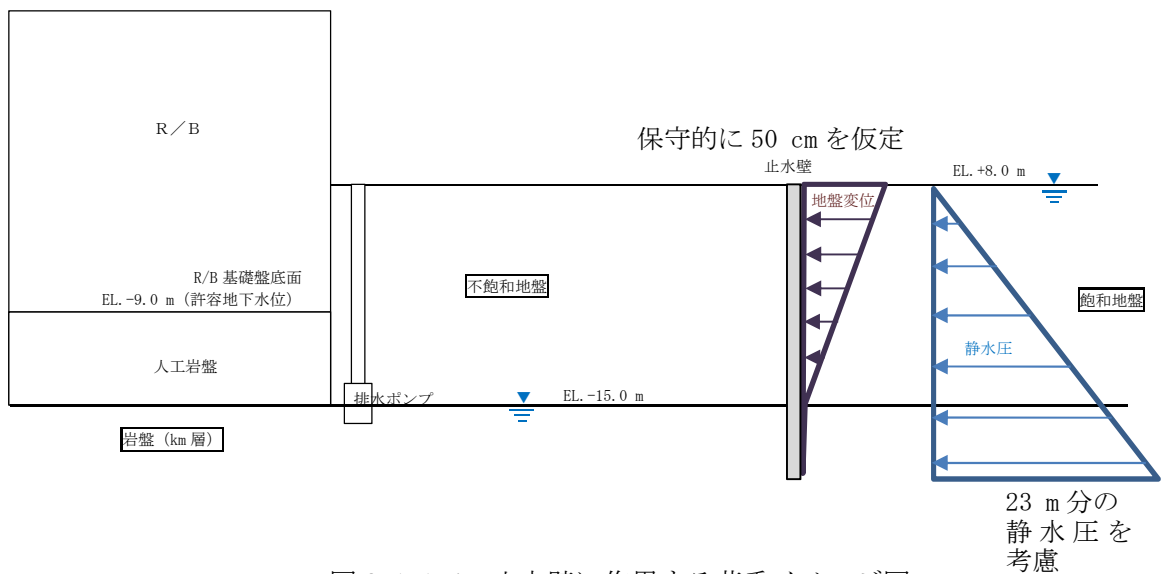
図 2. 1. 1-4 止水壁に作用する荷重イメージ図
