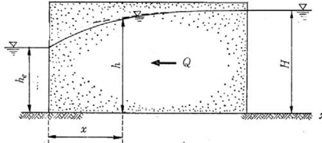
図 2.1.1-15 1次元定常浸透流地盤モデル
