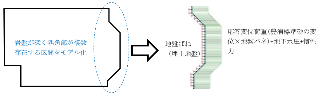
図 2.1.1-12 縦断面の応答変位法モデル図
