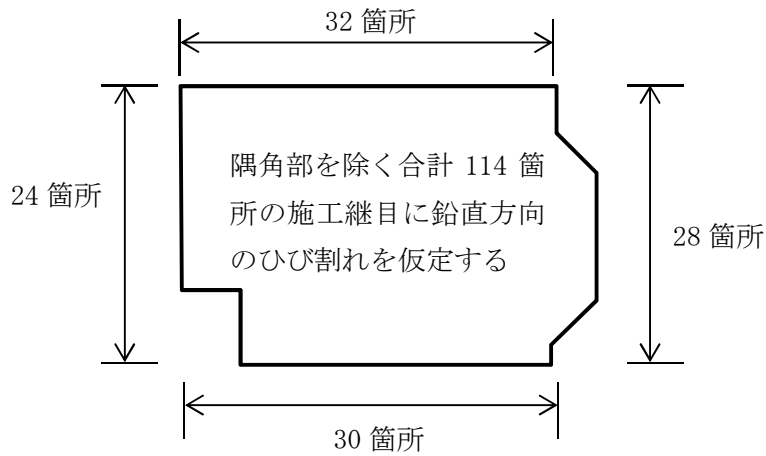
図 2.1.1-11 止水壁縦断面の直線部に仮定する鉛直方向ひび割れ
